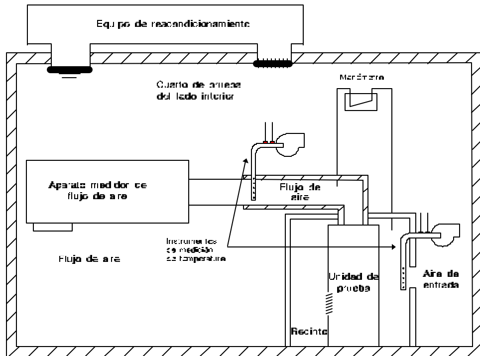
FIGURA 3. Calorímetro aire-entalpía
