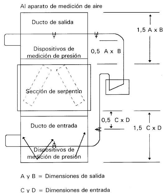
FIGURA 8. Medición de caída de presión estática del aire para una sección de serpentín sin ventiladores
