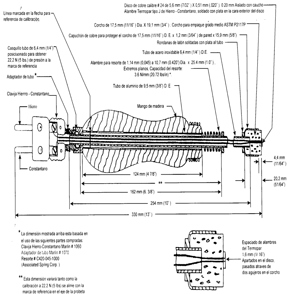
Figura 13. Probeta para Medición de Temperatura.
