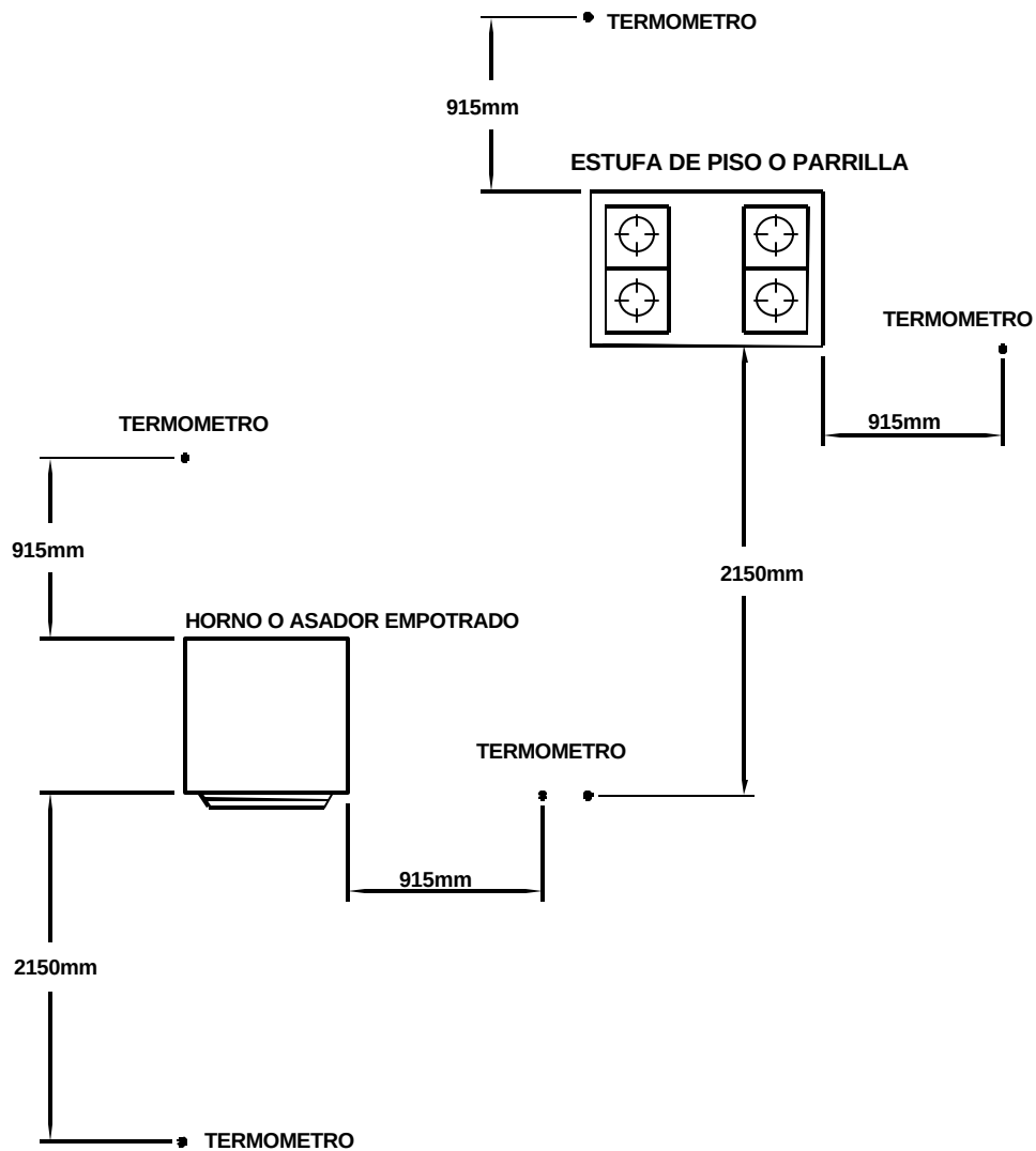
Figura 11.- Localización de termómetro para determinar temperatura ambiente.
