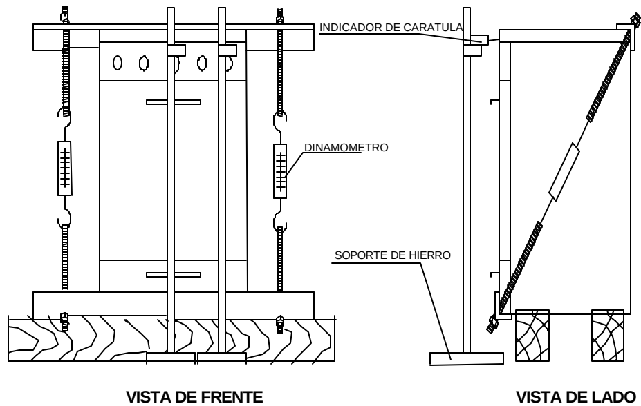
Figura 1.- Pruebas de resistencia a fuerzas diagonales del frente hacia atrás.
