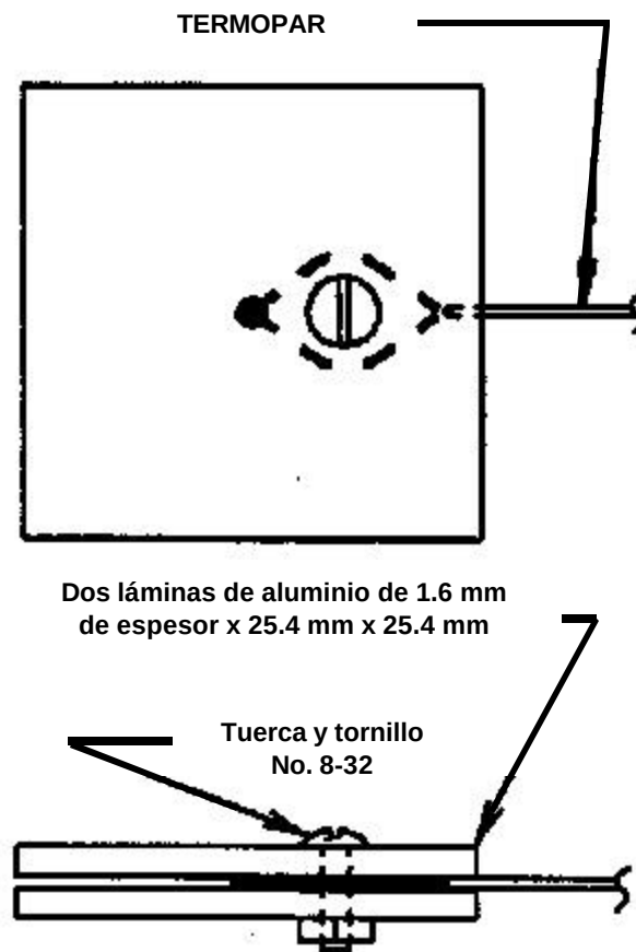
Figura 14. Arreglo para protección de termopares Tipo J con unión de gota.
