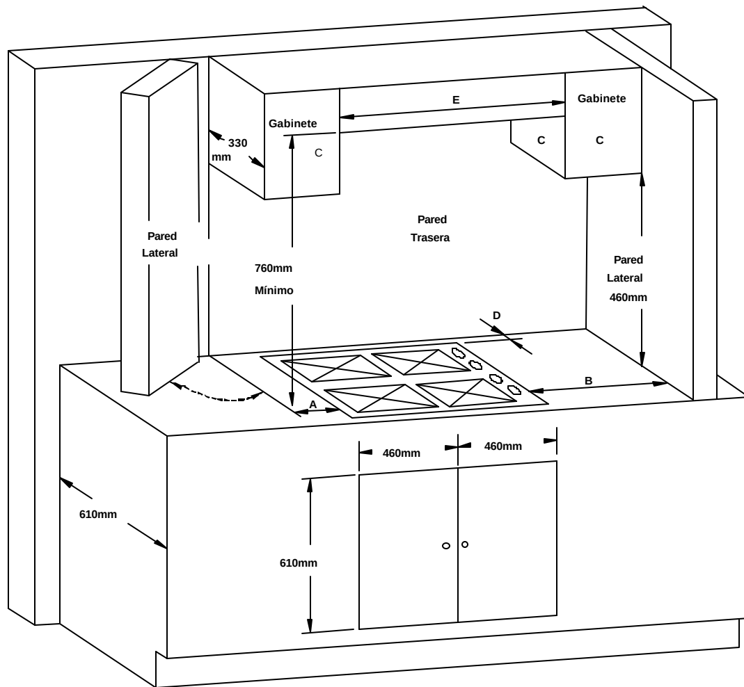
Figura 9.- Estructura para prueba de estabilidad de flamas de parrillas empotradas y asadores de superficie.
