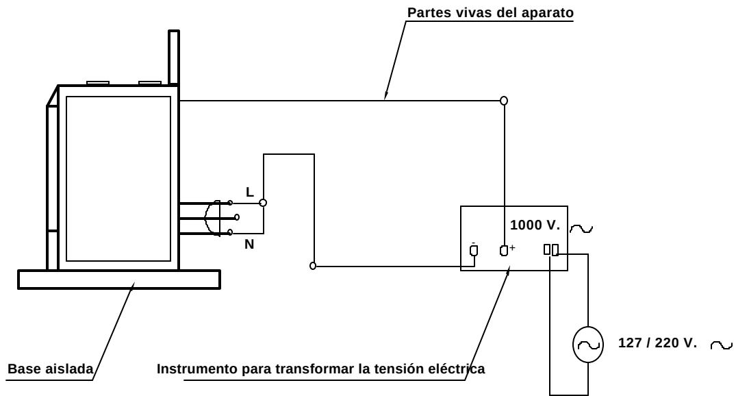
Figura 5.- Circuito de prueba para la rigidez dieléctrica.
