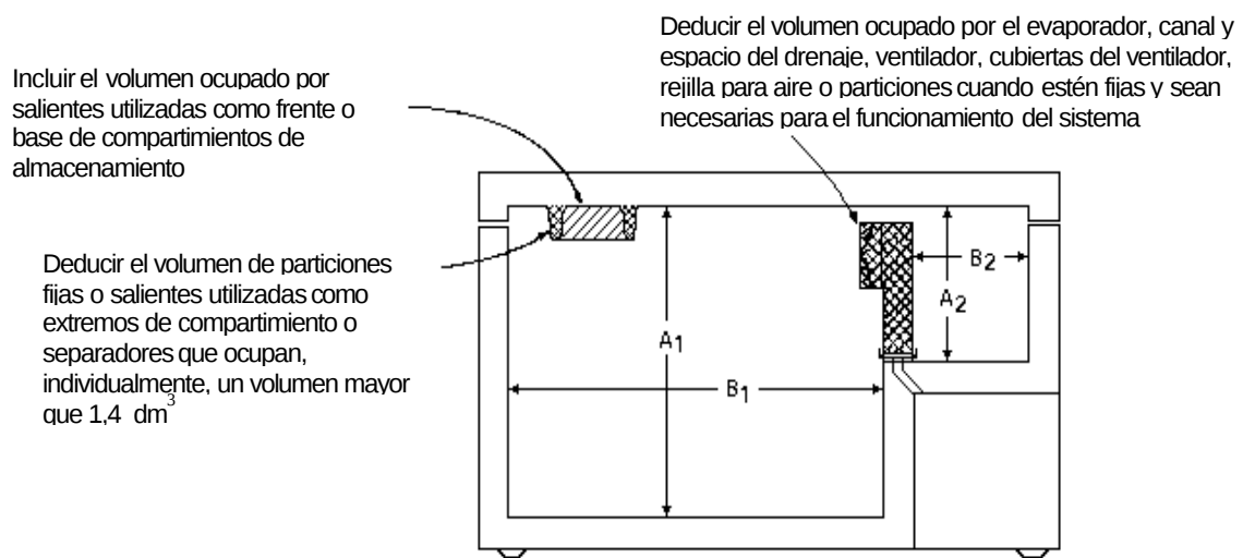
Figura 22. Congelador horizontal
