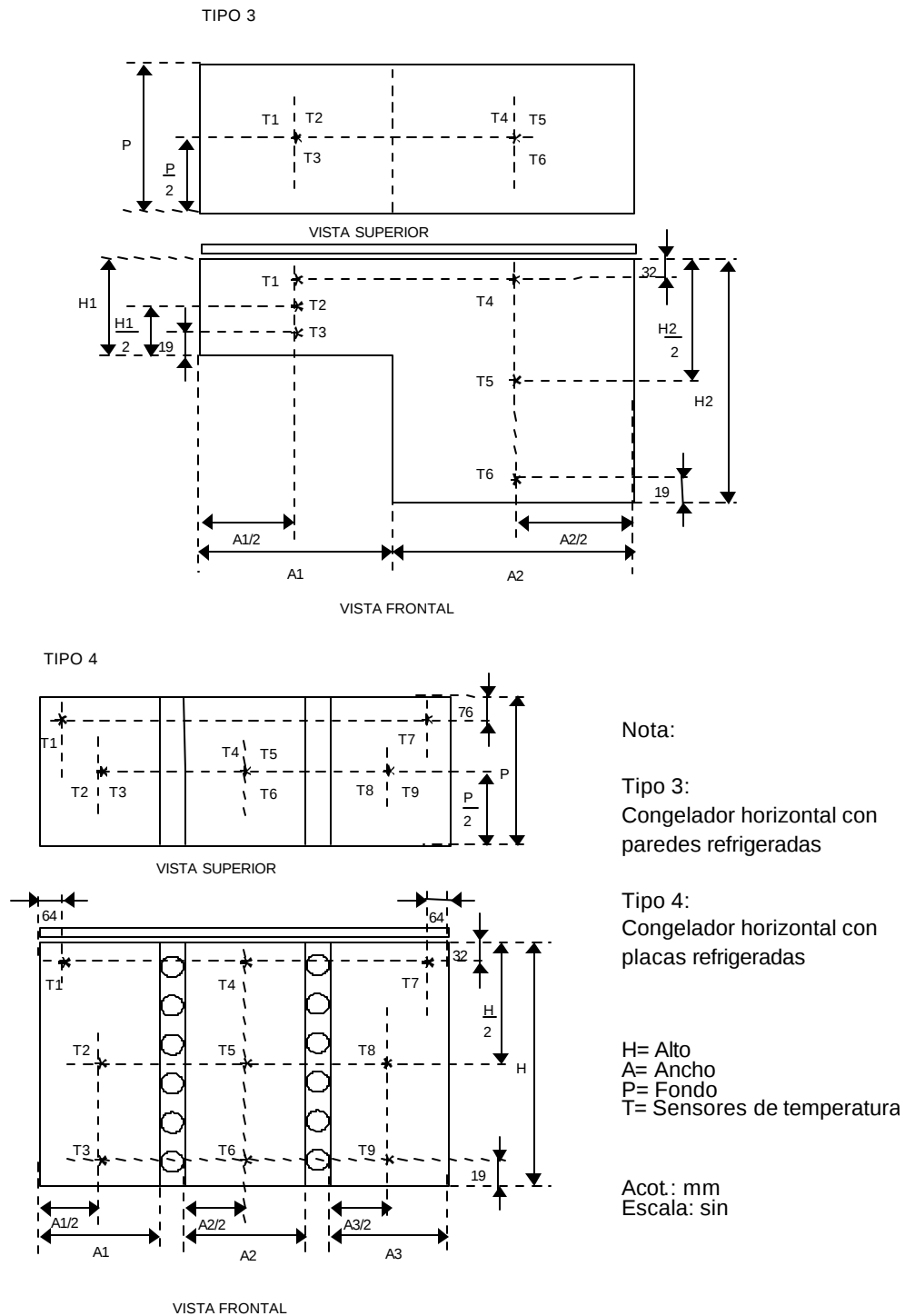
Figura 3. Colocación de sensores de temperatura en congeladores horizontales
