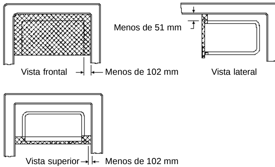
Figura 13. Deducciones de la puerta del evaporador
