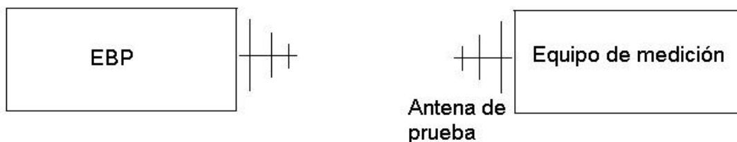
Figura 3. Configuraciones básicas para mediciones del método opcional
