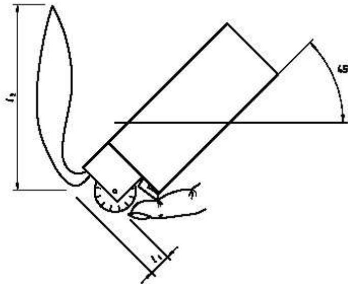
Figura 5: Medición de altura de flama para la prueba de flameo descrita en 7.2.3
