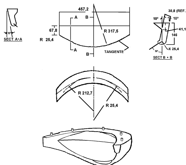
FIGURA 2.- Bloque metálico patrón usado en la prueba de resistencia de la ceja al desmontaje del rin
