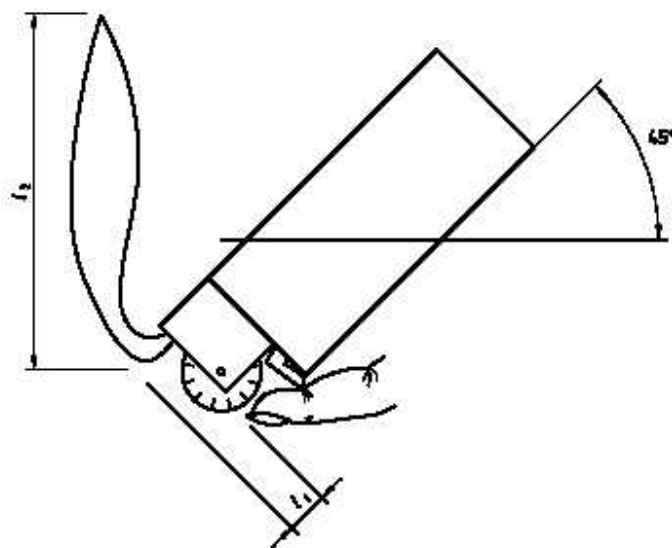
FIGURA 5: Medición de altura de flama para la prueba de flameo descrita en 7.2.2
