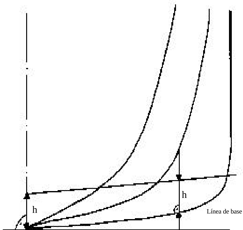
Figura 3: Definición de los límites de los tanques de carga a efectos del párrafo 7)
