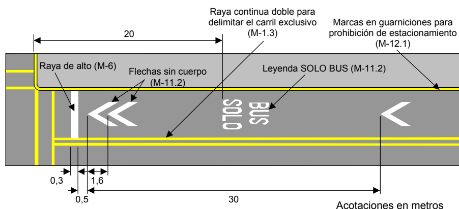
FIGURA 18.- Marcas para delimitar un carril en contrasentido
