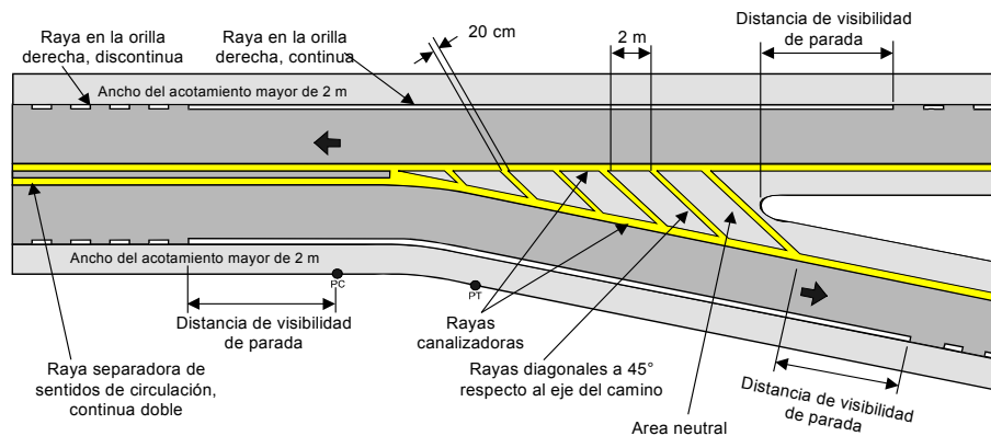
ANCHO DE CALZADA MAYOR DE 6,5 m
