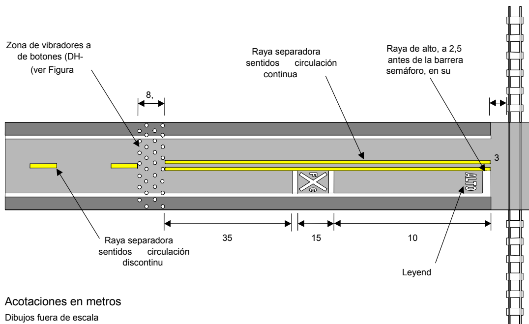
FIGURA 10.- Ubicación de vibradores para cruces de ferrocarril a nivel
