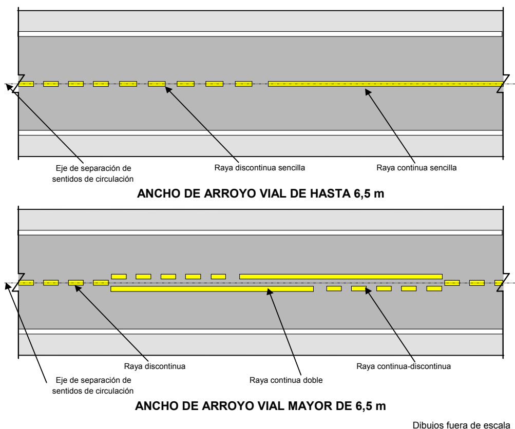
FIGURA 1.- Ubicación de la raya separadora de sentidos de circulación
