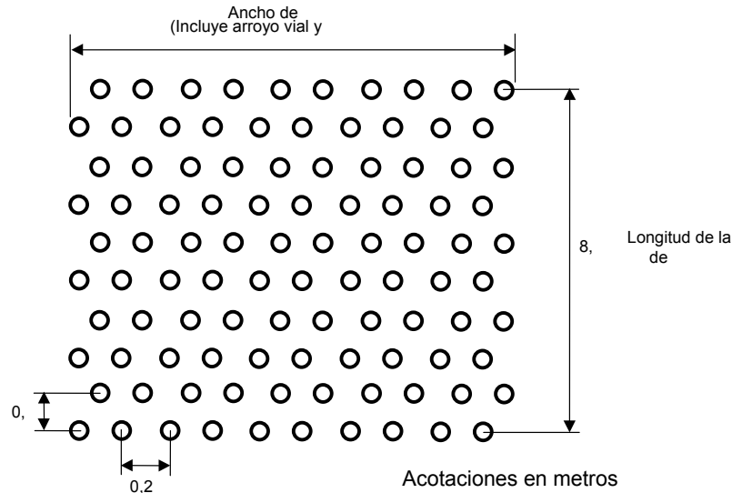
FIGURA 12.- Distribución de los botones (DH-3) en la zona de vibradores
