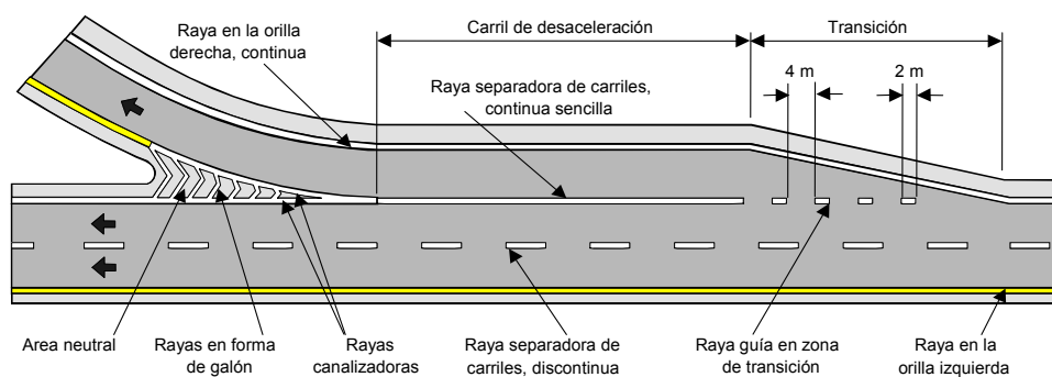
FIGURA 5.- Diversos tipos de rayas y marcas en el pavimento en aproximaciones de intersección
