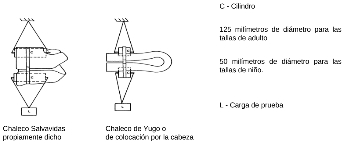
Figura 1.- Disposición de la prueba de resistencia del cuerpo del chaleco salvavidas
