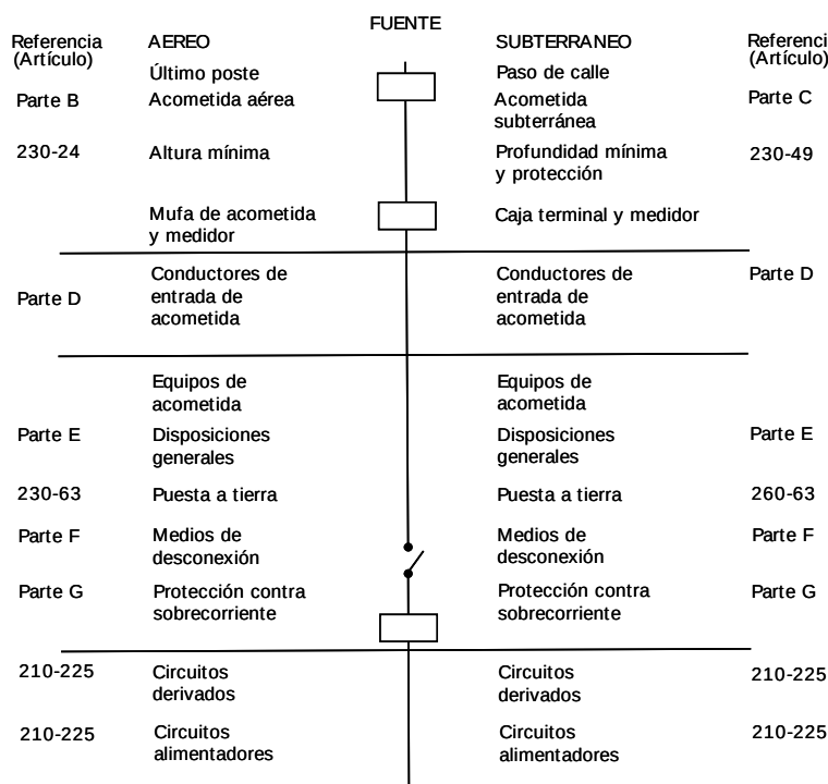
FIGURA 230-1.- Acometidas
