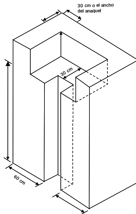
FIGURA 410-8.- Espacio de almacenamiento del clóset
