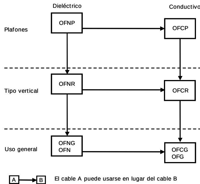
FIGURA 770-53. Jerarquía de sustitución de cables
