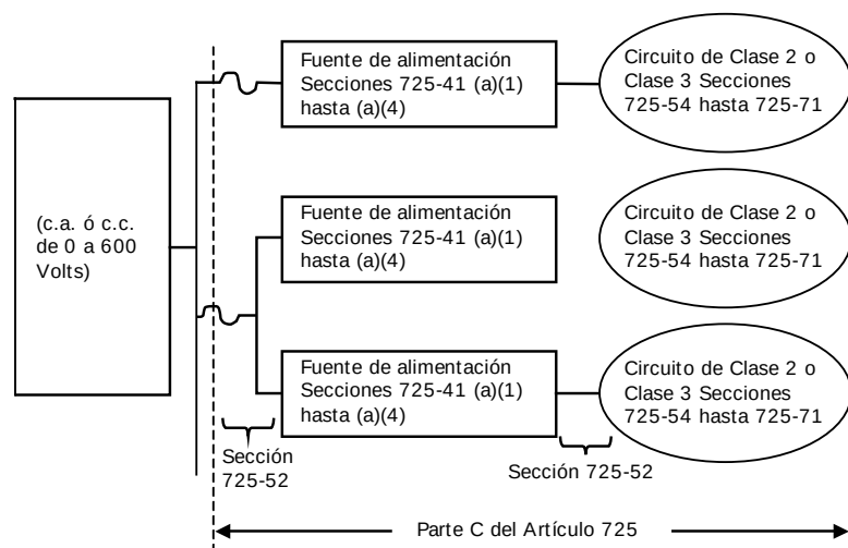
FIGURA 725-41.- Circuitos Clase 2 y Clase 3
