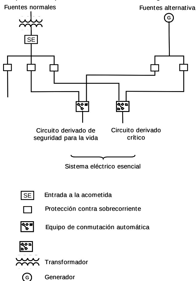
FIGURA 517-41(a).- Sistema eléctrico pequeño en lugares para enfermerías y áreas de atención limitada
