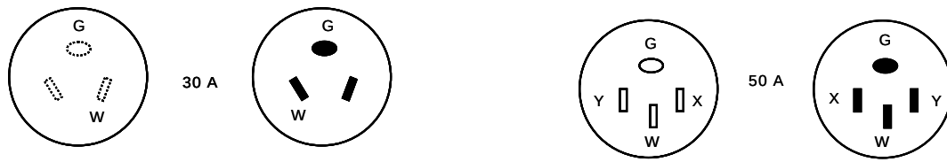
FIGURA 552-44(c).- Configuraciones para receptáculos y clavijas del tipo con puesta a tierra utilizados para cordones para alimentar vehículos de recreo y sus estacionamientos
