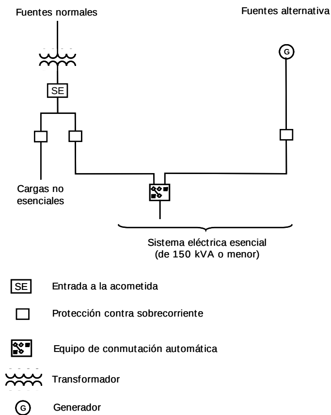
FIGURA 517-41(c) Sistema eléctrico pequeño en lugares para enfermería y áreas de atención limitada (con un solo desconectador de transferencia)
