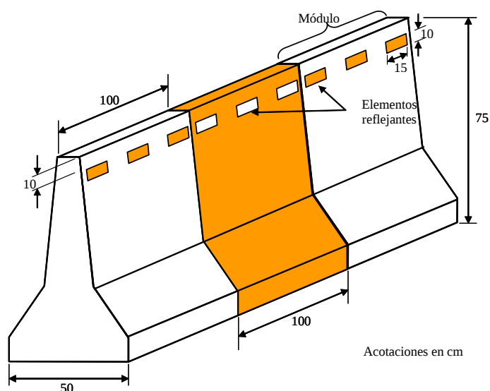
FIGURA 2.- Colocación de las barreras fijas en serie
