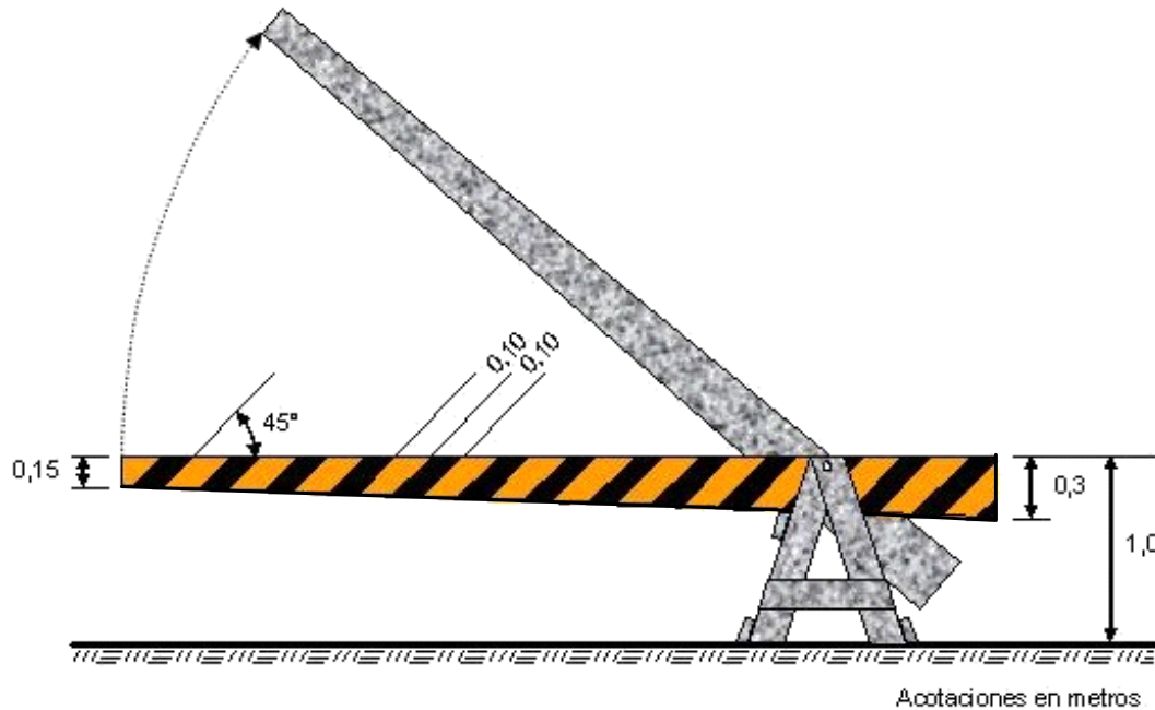
FIGURA 1.- Barrera levadiza
