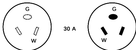
FIGURA 552-44(c).- Configuraciones para receptáculos y clavijas del tipo con puesta a tierra utilizados para cordones para alimentar vehículos de recreo y sus estacionamientos
