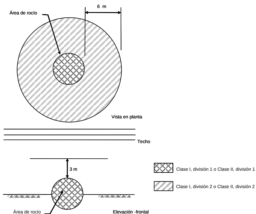
FIGURA 516-2 (b)(1).- Áreas Clase I o Clase II División 2, adyacentes a una operación de rociado abierto
