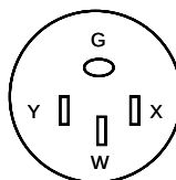
FIGURA 552-44(c).- Configuraciones para receptáculos y clavijas del tipo con puesta a tierra utilizados para cordones para alimentar vehículos de recreo y sus estacionamientos
