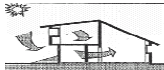
Fig. 3 Esquema del funcionamiento de las trampas de calor.
