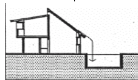
Fig. 6 Formas de captación y almacenamiento pluvial.
