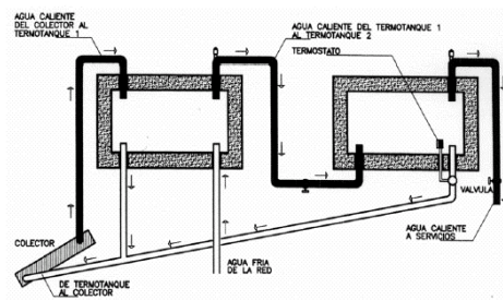
Fig. 2 Esquema de interconexión de colectores solares.
