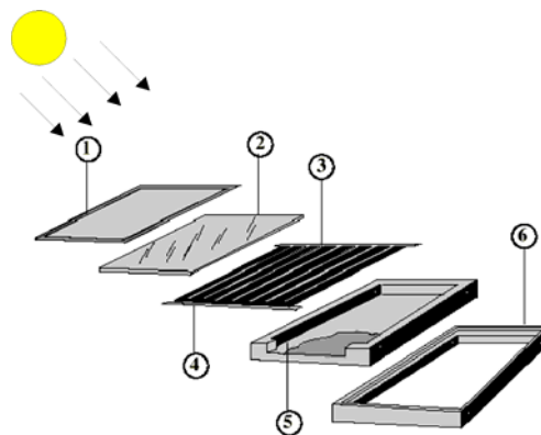
Fig. 1 Esquema transversal de colector solar
