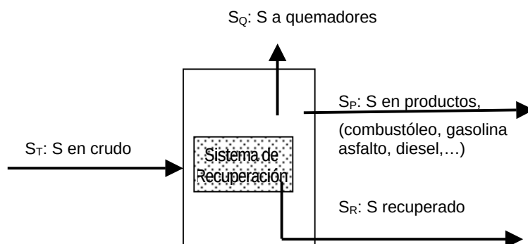
Figura 1. Balance de azufre de una refinería
