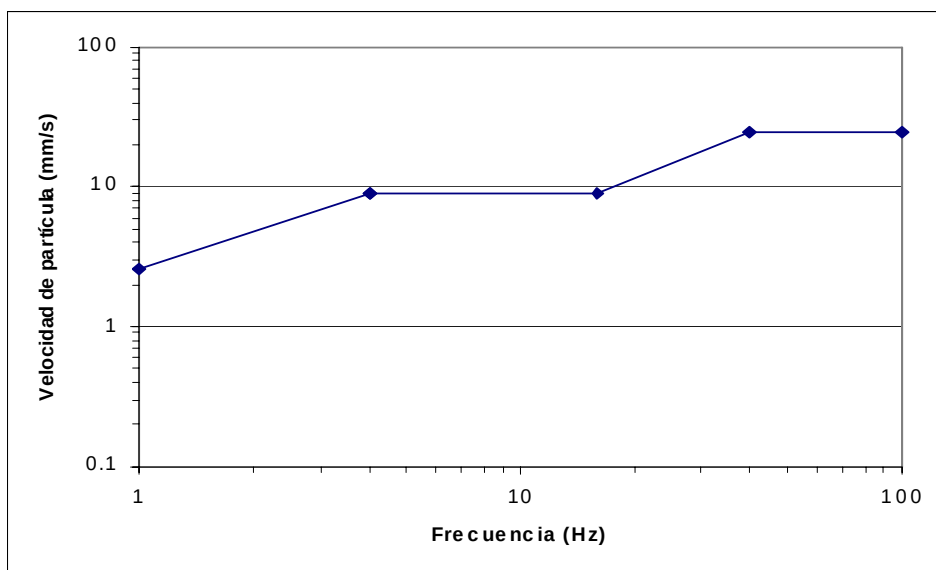
Figura 1, Curva límite de referencia
