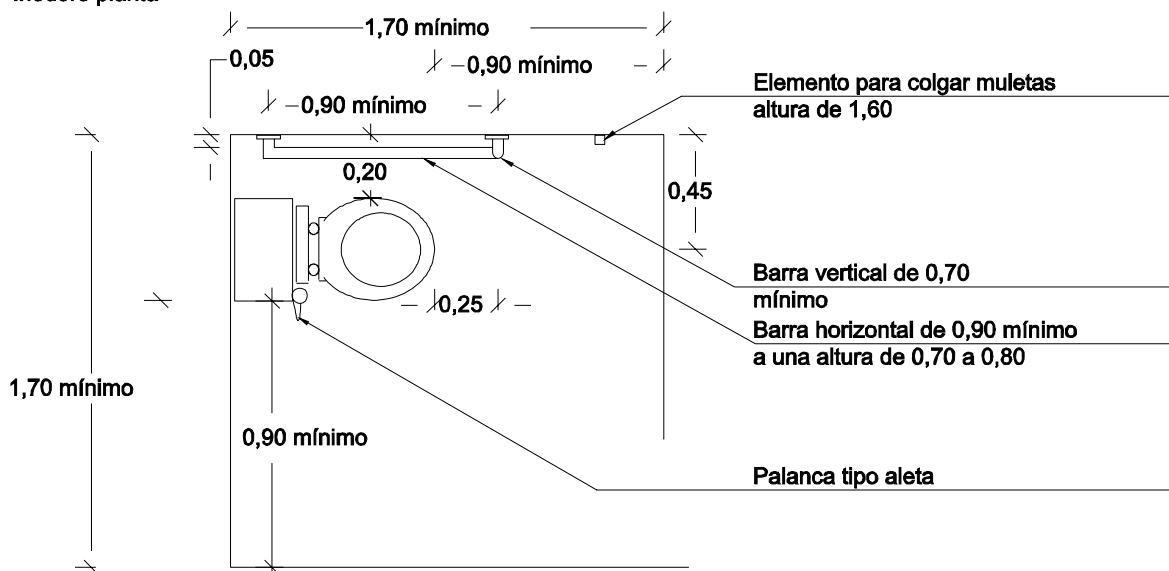
Inodoro planta
