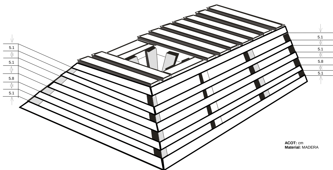
FIGURA 1 - Especificaciones de las trampas de madera.
