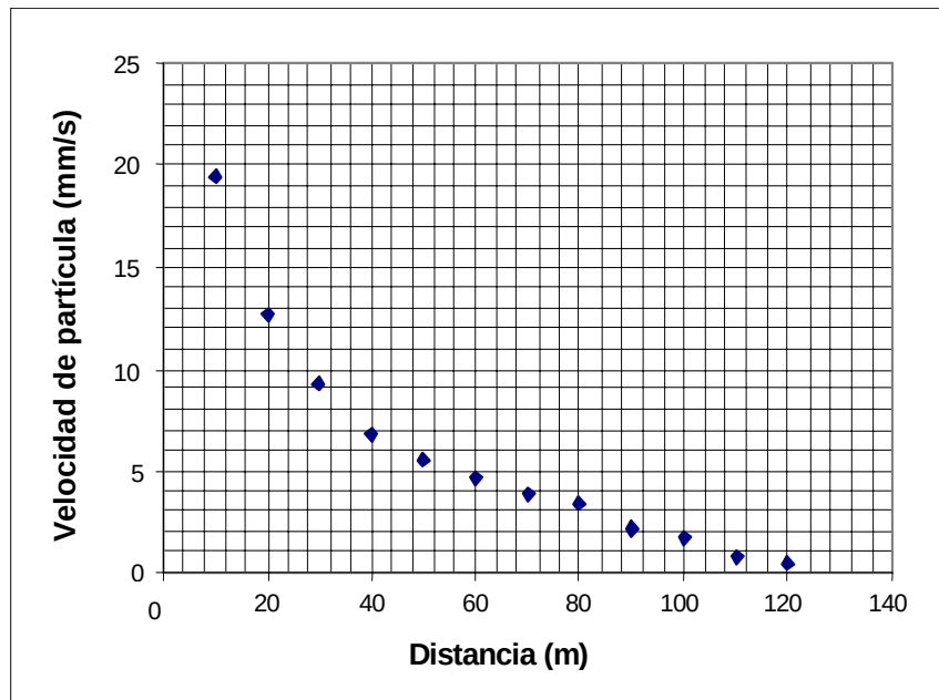
Figura 2, Velocidad máxima de partícula vs. Distancia
