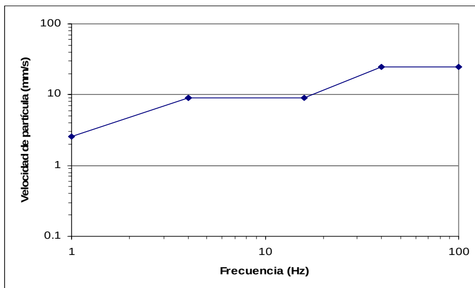
Figura 1, Curva límite de referencia
