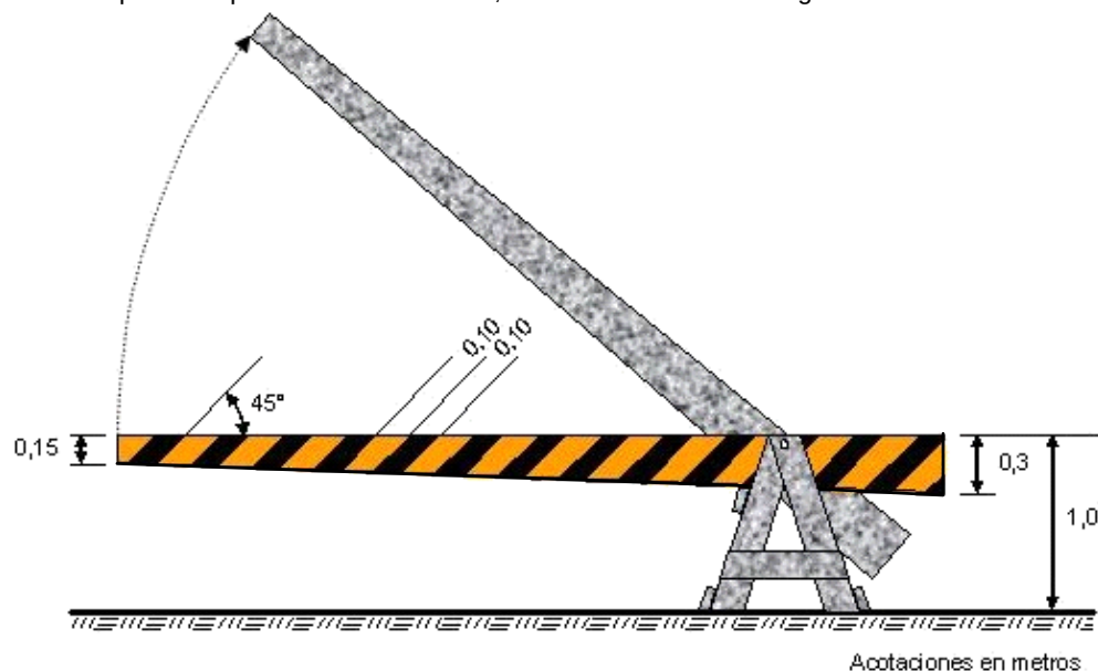
FIGURA 1.- Barrera levadiza
