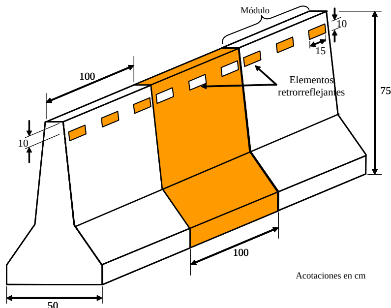
FIGURA 2.- Colocación de las barreras fijas en serie
