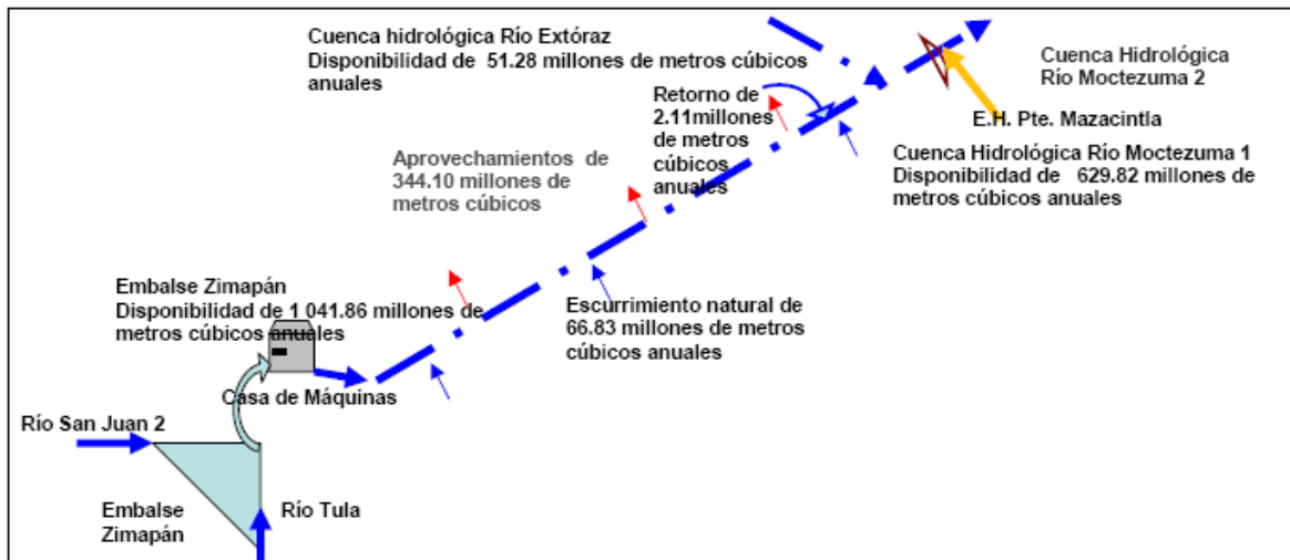
Figura 5.5 Diagrama de balance Cuenca Hidrológica Río Moctezuma 1.
