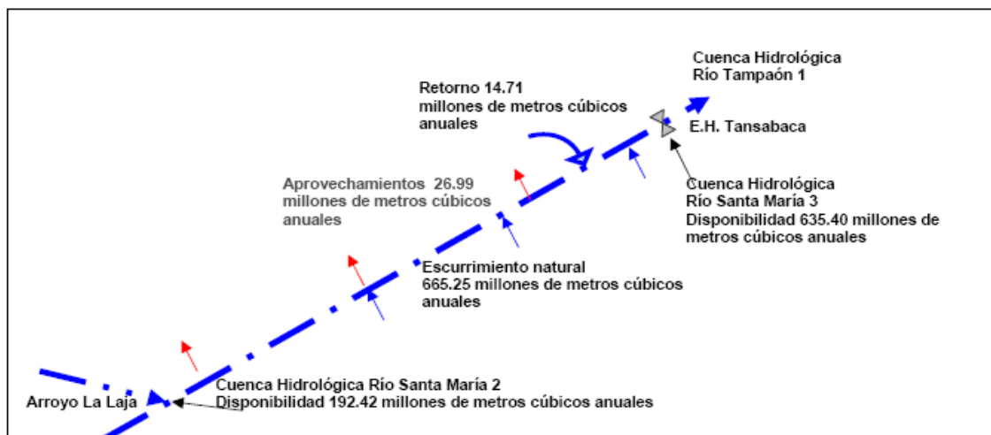
Figura 5.3 Diagrama de la Cuenca Hidrológica Río Santa María 3.
