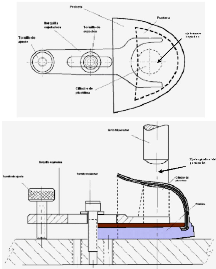
Figura 3. Posición de la probeta en el equipo de prueba de impacto a la puntera
