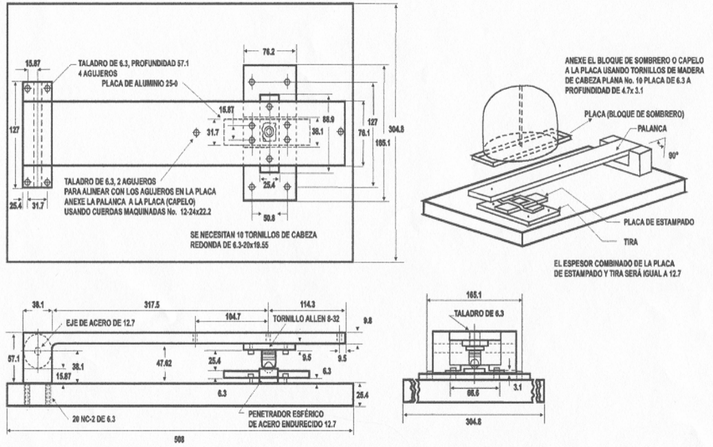
Figura 1. Montaje Brinell para prueba de impacto
