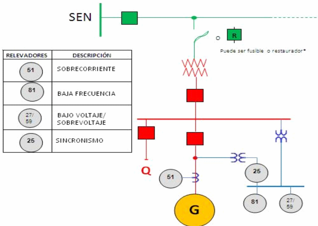
Figura No. 2 Diagrama básico de interconexión
