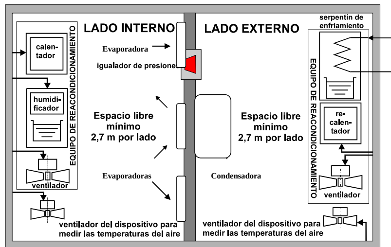
Figura 2. Calorímetro de cuarto tipo calibrado
