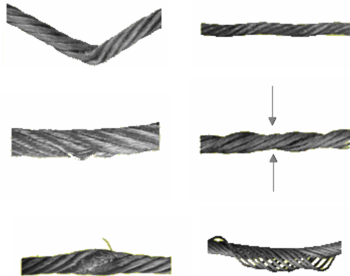
Figura 9 Ejemplos de condiciones inseguras en cables
