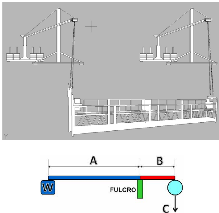
Figura 7 Contrapesos en andamios suspendidos
