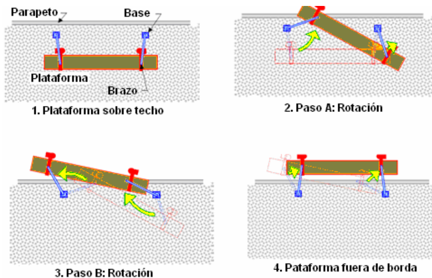
Figura 8 Instalación de la hamaca o plataforma
