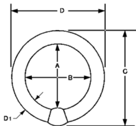
Figura B4.- Dimensiones de la lámpara circular con base G10q
