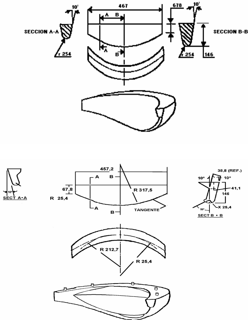
Figura 2.- Bloques metálicos patrón usados en la prueba de resistencia de la ceja al desmontaje del rin.
