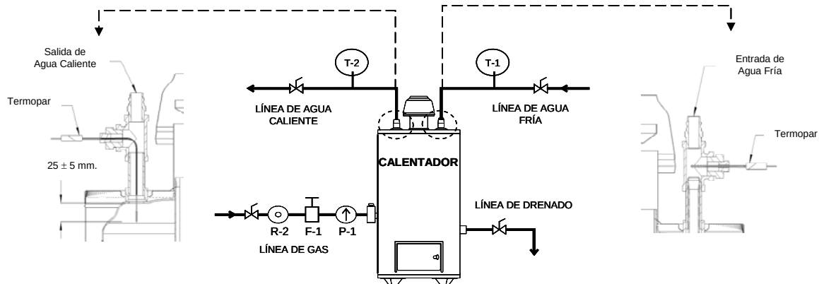
FIGURA 1A.- Esquema de tubería e instrumentación para la prueba de eficiencia térmica en calentadores de agua de almacenamiento para uso doméstico y comercial.
