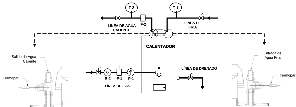
FIGURA 2A.- Esquema de tubería e instrumentación para la prueba de eficiencia térmica en calentadores de agua de rápida recuperación para uso doméstico y comercial.
