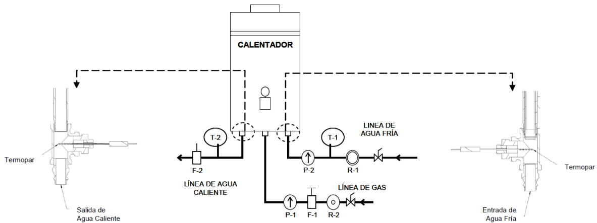
FIGURA 3A.- Esquema de tubería e instrumentación para la prueba de eficiencia térmica en calentadores de agua instantáneo para uso doméstico y comercial.
