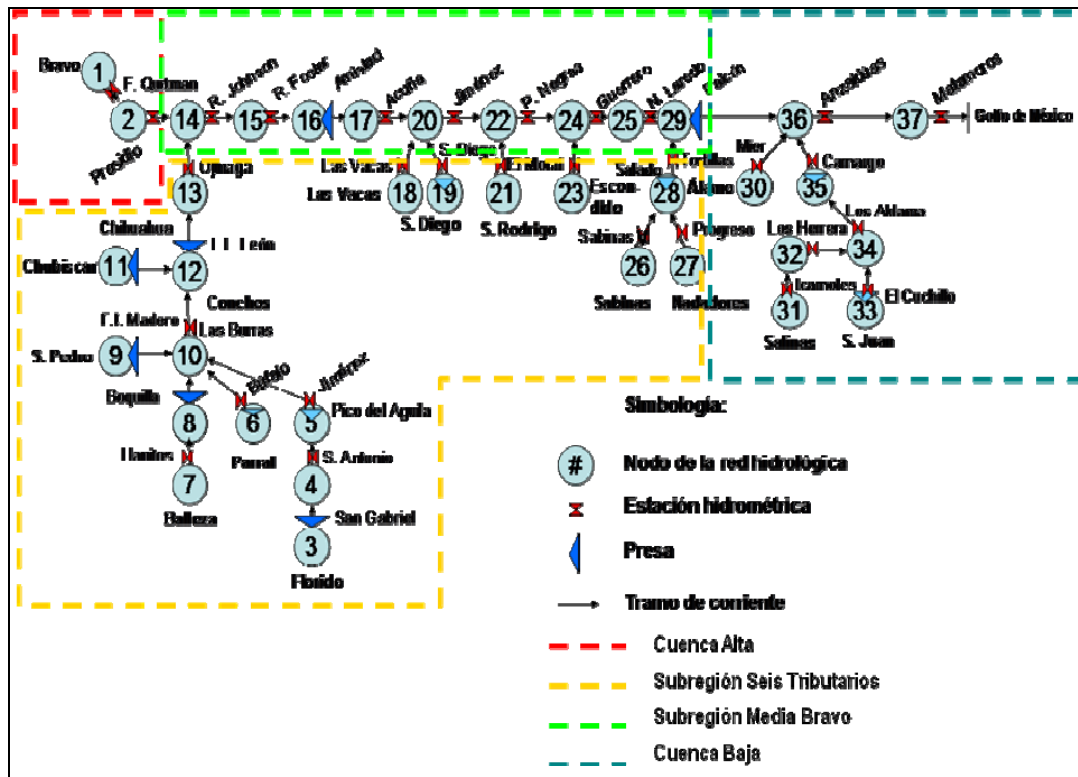
Figura 9. Diagrama unifilar de la Región Hidrológica número 24 Bravo-Conchos para cálculo de disponibilidad
