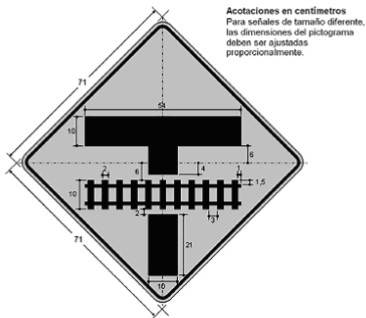
FIGURA B4.- SP-35C "Cruce con vía férrea e intersección en T secundaria" de 71 x 71 cm
