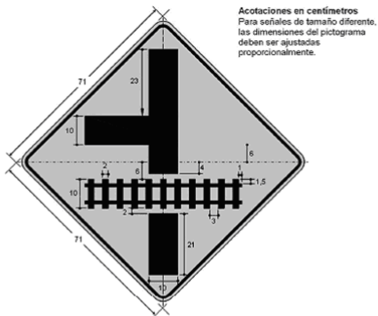
FIGURA B3.- SP-35B "Cruce con vía férrea a e intersección en T principal" de 71 x 71 cm
