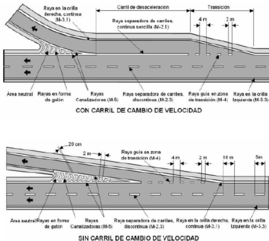
FIGURA 7.- Rayas separadoras de carriles, rayas guía en zonas de transición, rayas canalizadoras y rayas en la orilla del arroyo vial
