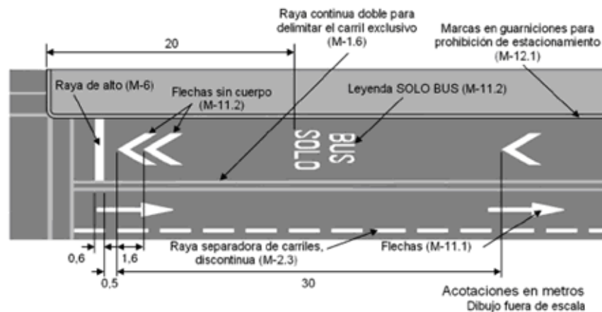
FIGURA 4.- Marcas para delimitar un carril en contrasentido.
