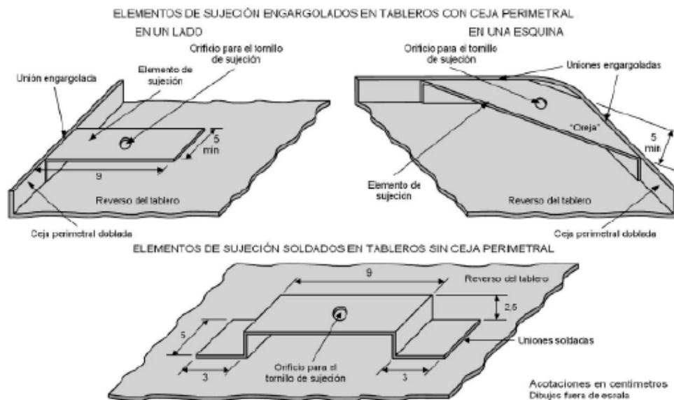
FIGURA 35.- Elementos de sujeción para señales bajas
