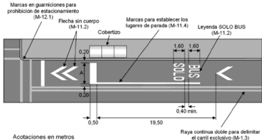
FIGURA 21.- Marcas para establecer lugares de parada en un carril en contrasentido
