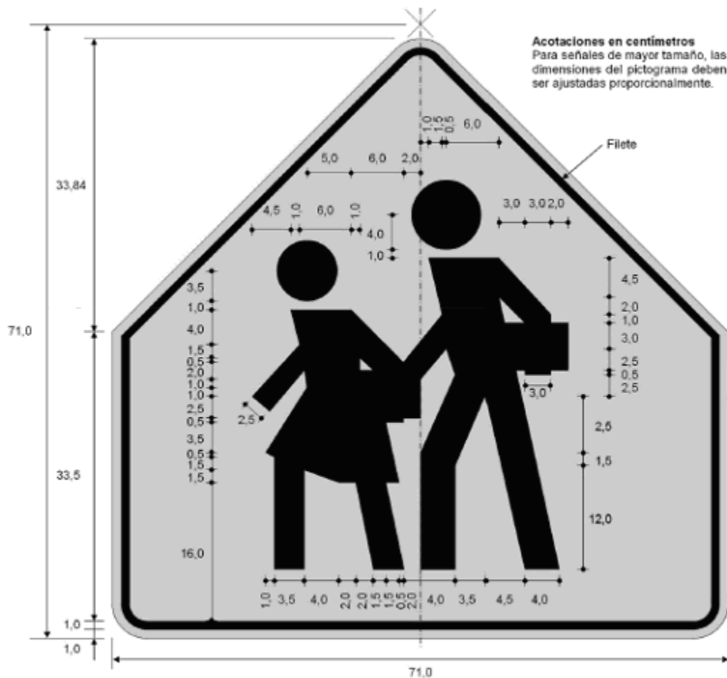
FIGURA 28.- Señal preventiva SP-33 "Escolares" de 71 x 71 cm
