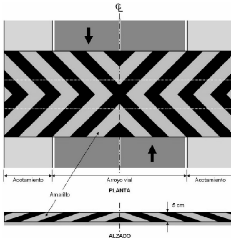
FIGURA 27.- Color de los reductores de velocidad (RV)
