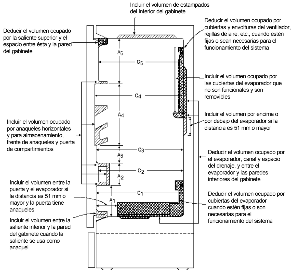
Figura 19. Congelador vertical
