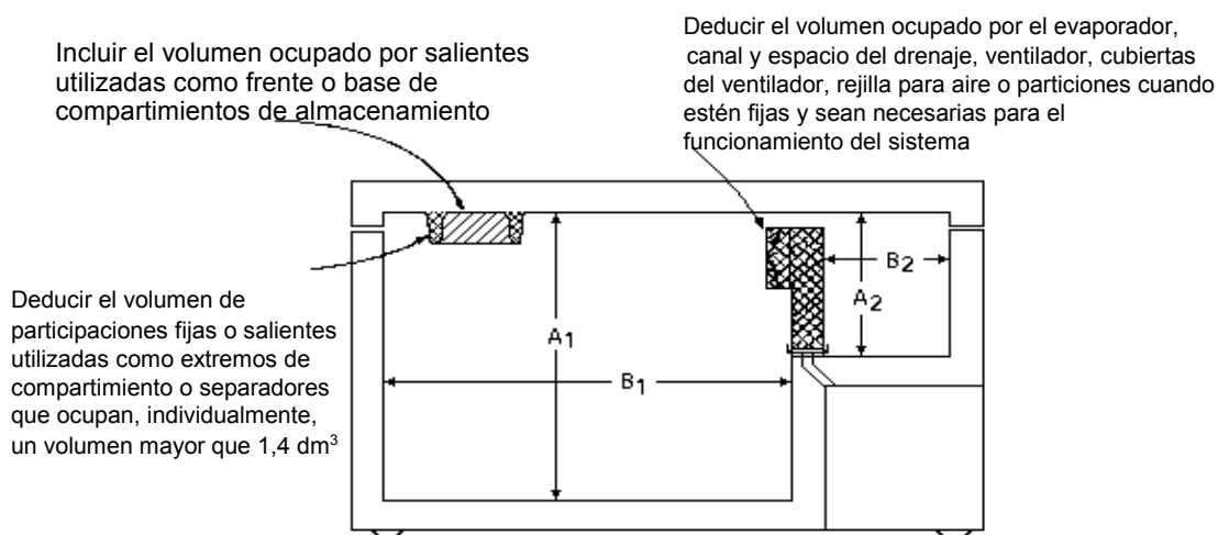
Figura 22. Congelador horizontal
