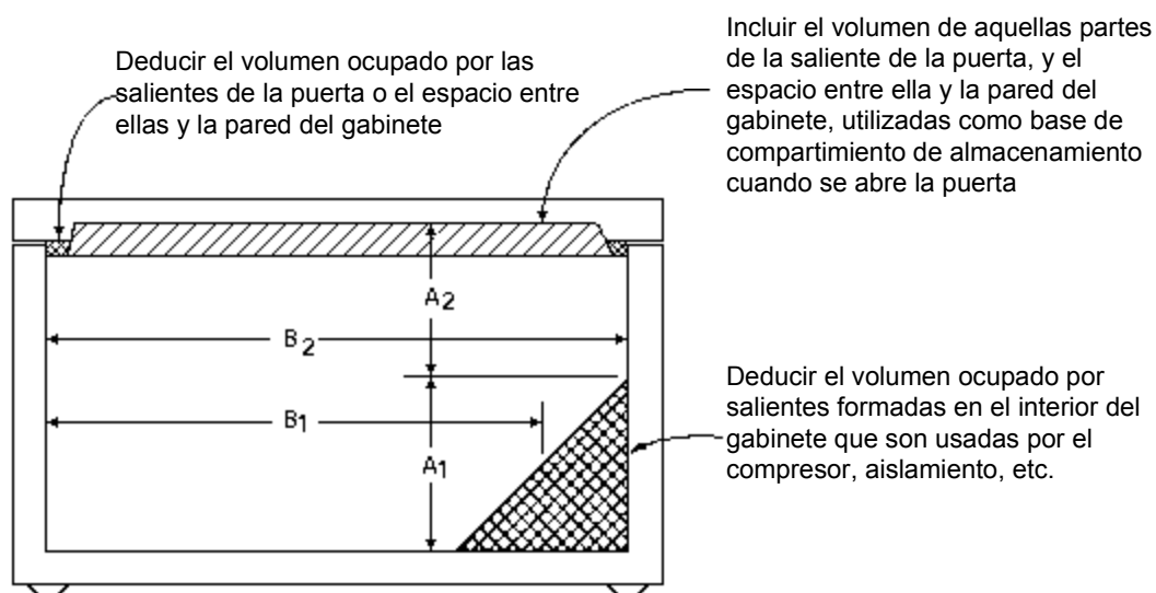
Figura 21. Congelador horizontal
