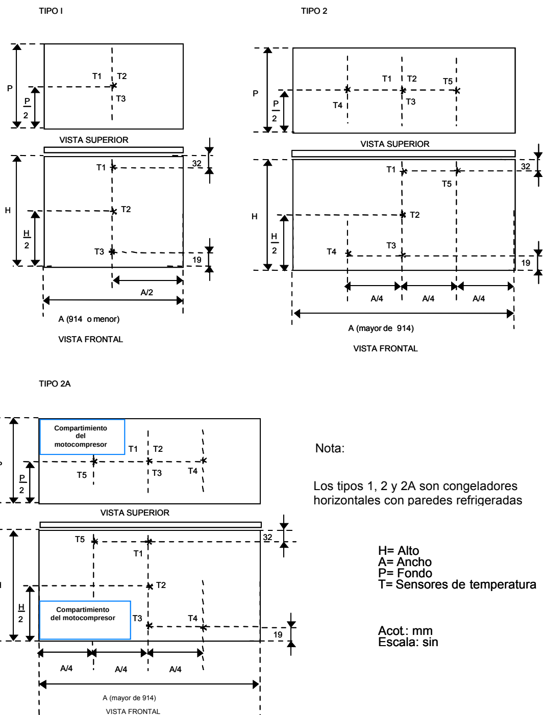
Figura 2. Colocación de sensores de temperatura en congeladores horizontales
