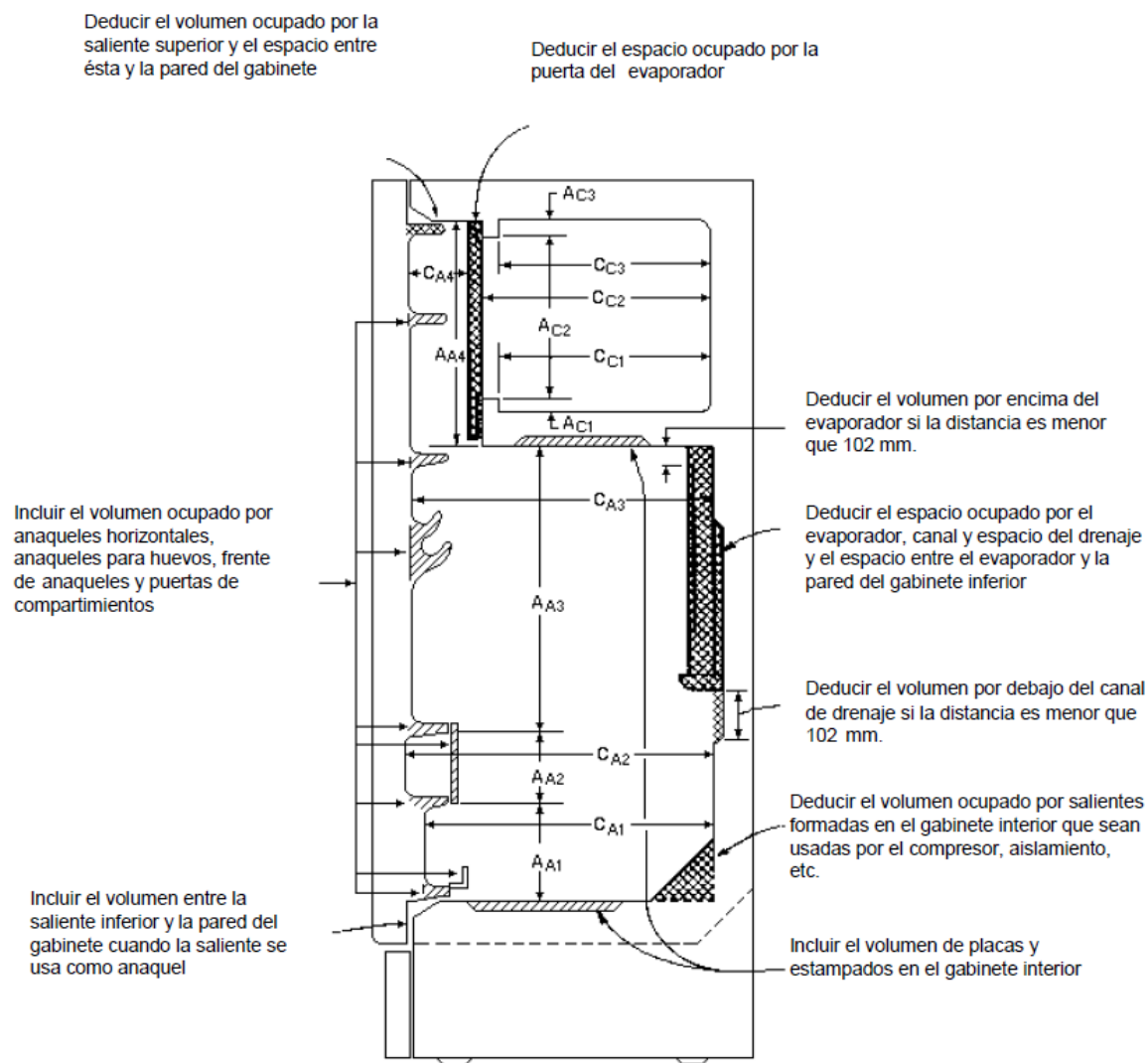
Figura 7. Refrigerador convencional
