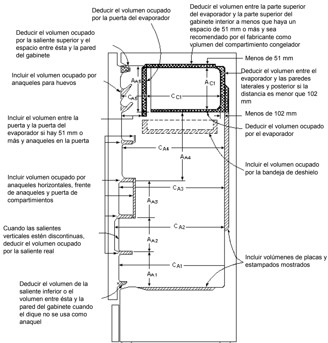
Figura 6. Refrigerador convencional
