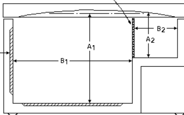
Figura 20. Congelador horizontal
