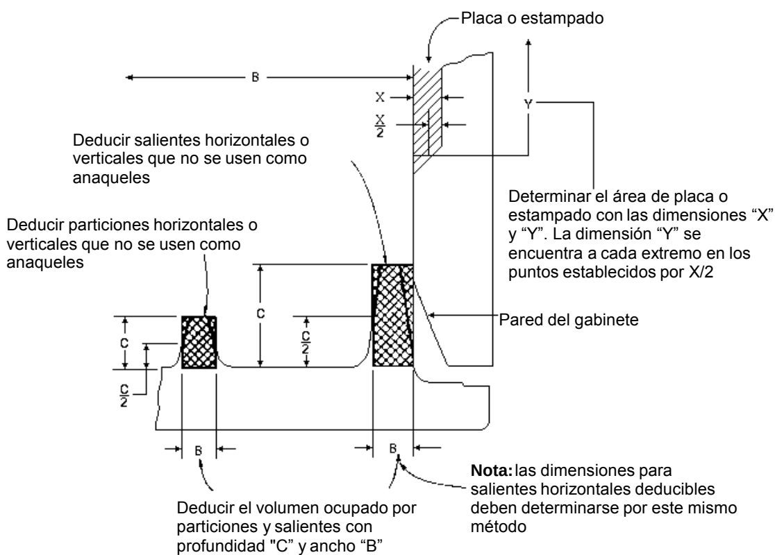
Figura 23. Saliente de la puerta y dimensiones lineales de la placa
