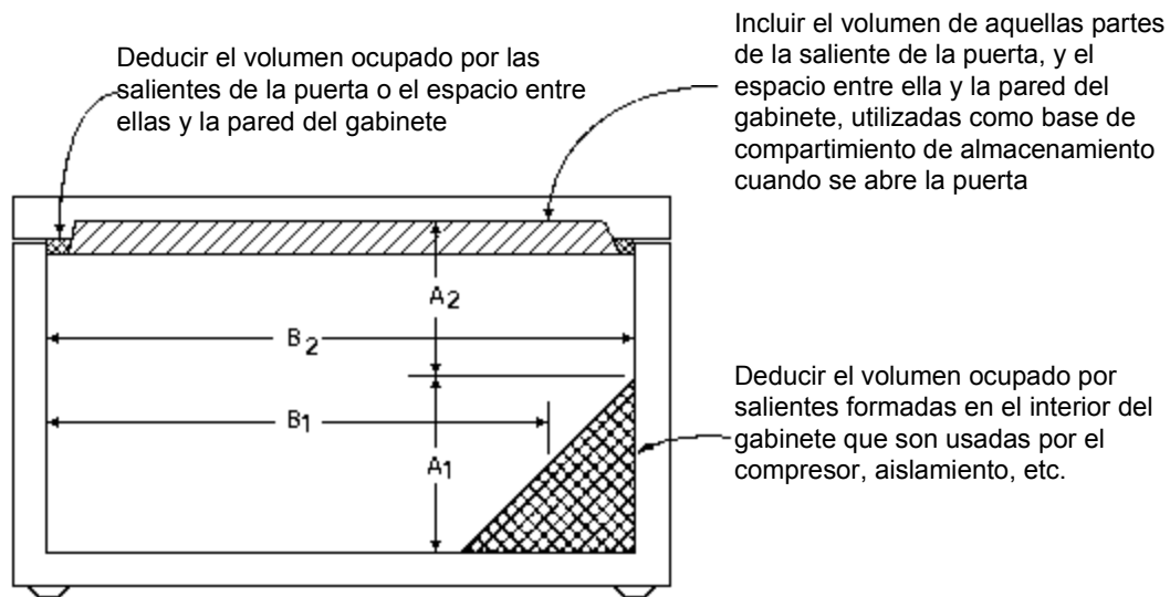
Figura 21. Congelador horizontal
