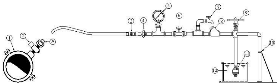
Figura 2. Esquema de prueba abrazadera/ sileta y válvula de inserción
