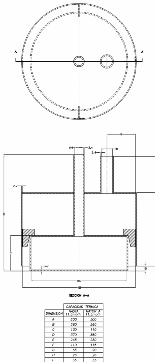
Figura 11. Prueba de combustión: Campana de recolección de gases de quemadores superiores
