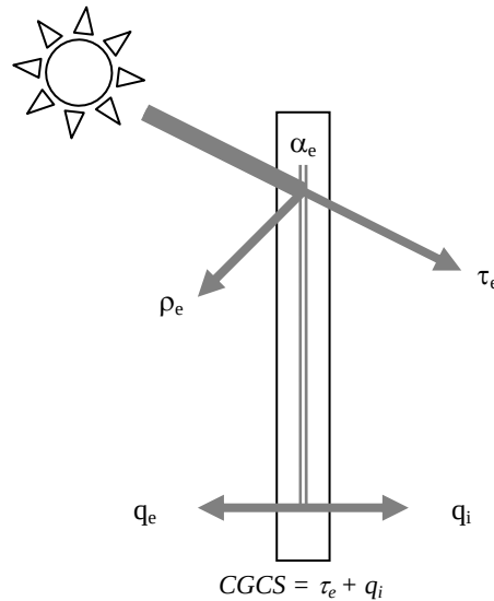
Figura A.1.- Comportamiento de la radiación solar a través de un vidrio
