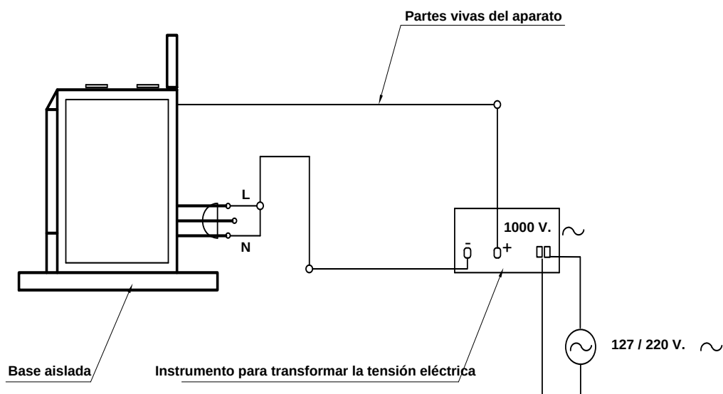
Figura 9. Circuito de prueba para aguante del dieléctrico a la tensión
