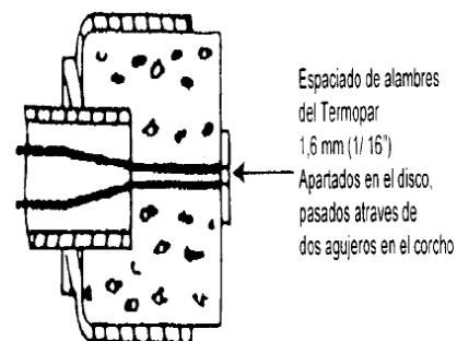
Figura 15. Probeta para medición de temperatura de superficies
