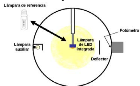
Figura G.1. Configuración de la esfera integradora 4\pi
