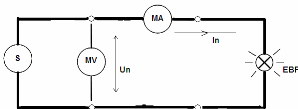
CIRCUITO DE MEDICION Y FUENTE DE ALIMENTACIÓN PARA DISTORSIÓN TOTAL DE ARMÓNICAS EN TENSIÓN Y CORRIENTE
