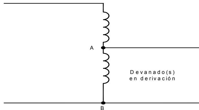
Figura 450-4.- Autotransformador
