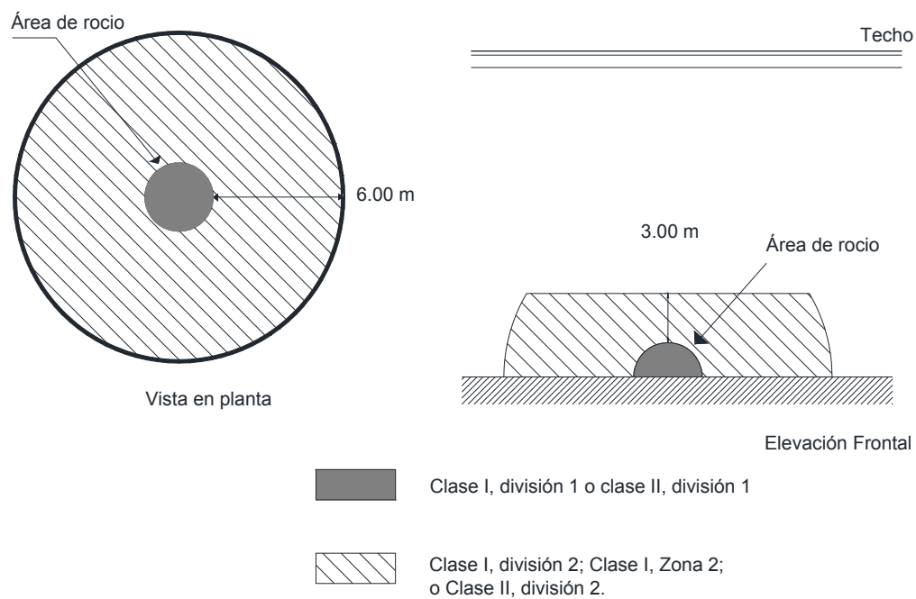
Figura 516-3(c)(1).- Clasificación eléctrica de las áreas para rociado abierto.
