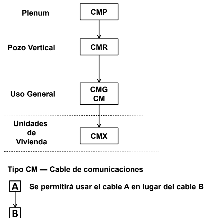
Figura 800-154.- Jerarquía de sustituciones de cables.
