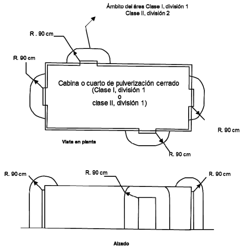
Figura 516-3(c)(4).- Áreas Clase I, División 2; Clase I, Zona 2 o Clase II, División 2 adyacentes a un recinto o una cabina de rociado encerrados
