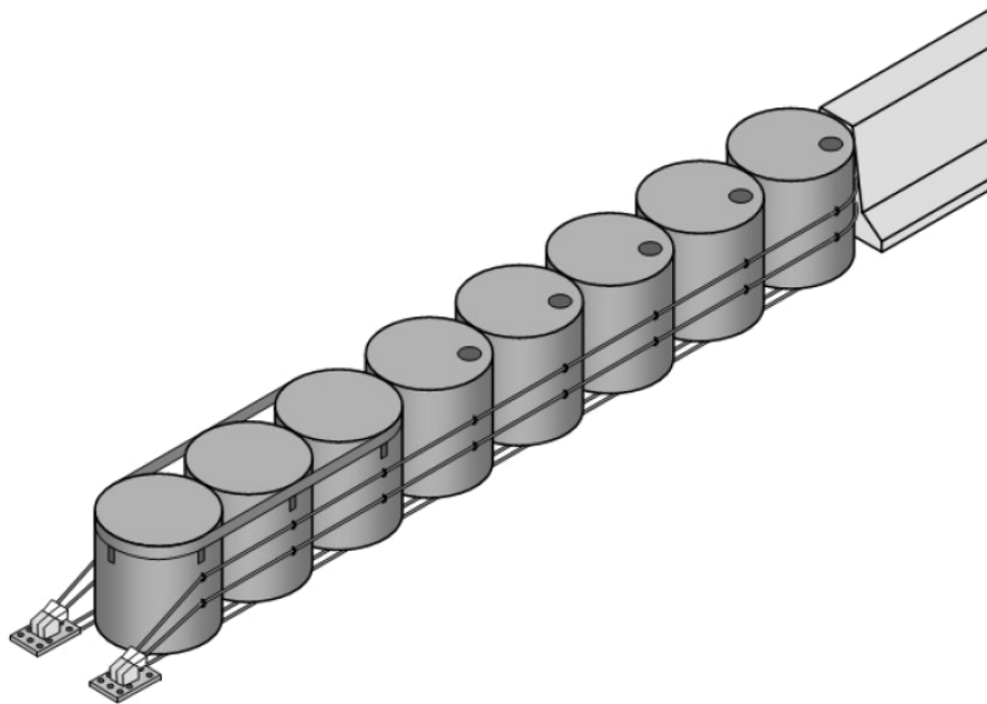
FIGURA 24.- Sección de amortiguamiento redireccionable – traspasable (OD-4.4.1/RT)
