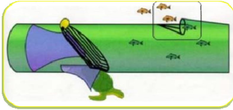
Figura D2 Dispositivo excluidor de peces "ojo de pescado" instalado en el bolso de la red, antes del dispositivo excluidor de tortugas.
