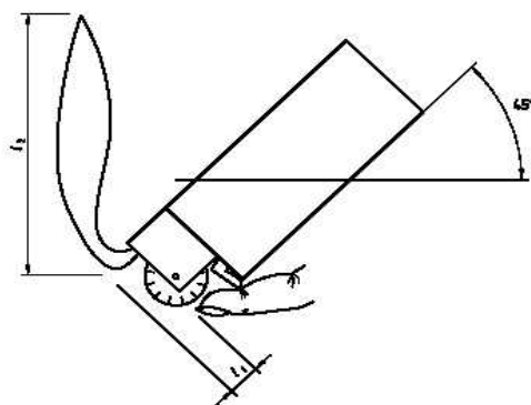
Figura 4: Medición de altura de flama para la prueba de flameo descrita en 7.2.3.2
