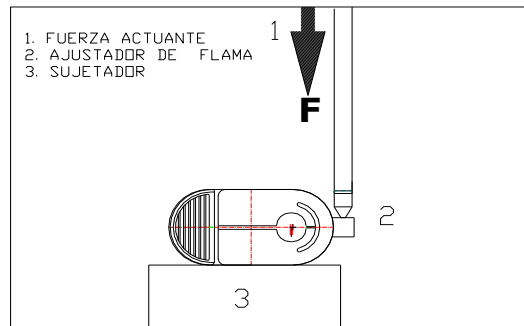
FIGURA 2: APLICACION DE LA FUERZA ACTUANTE PARA CONTROL DE LA FLAMA
