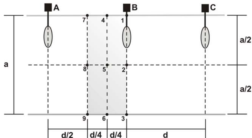
Figura C.1. Distribución unilateral
