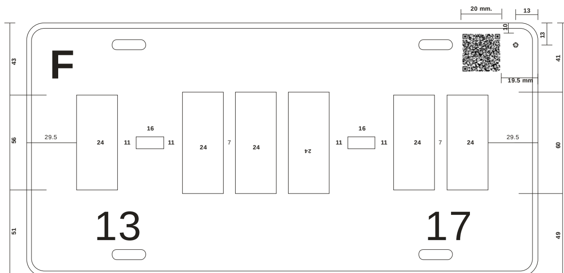
Figura 13 Separación de caracteres (letras y dígitos) placas con seis caracteres y guiones Placa para DEMOSTRACIÓN (Entidades Federativas)
