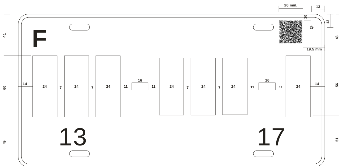
Figura 18 Separación de caracteres (letras y dígitos) placas con siete caracteres y guiones Placa para TRANSPORTE PRIVADO AUTOMÓVIL (Entidades Federativas)
