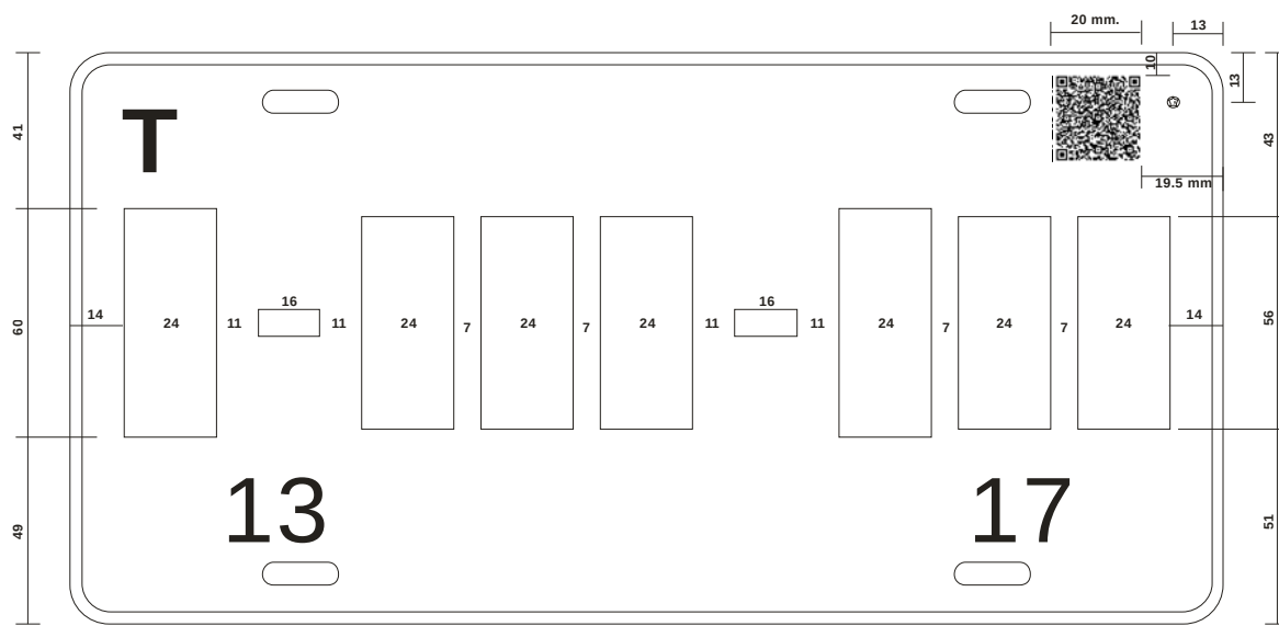
Acotaciones en milímetros El ancho de los caracteres debe ser de acuerdo a lo indicado en la figura Se incorpora la letra "T" y "F" según corresponda a la placa Las dimensiones del guión separador serán de 16 x 5.6 Figura 28 Separación de caracteres (letras y dígitos) placas con siete caracteres y guiones Placa para Remolque Público Local (Entidades Federativas)
