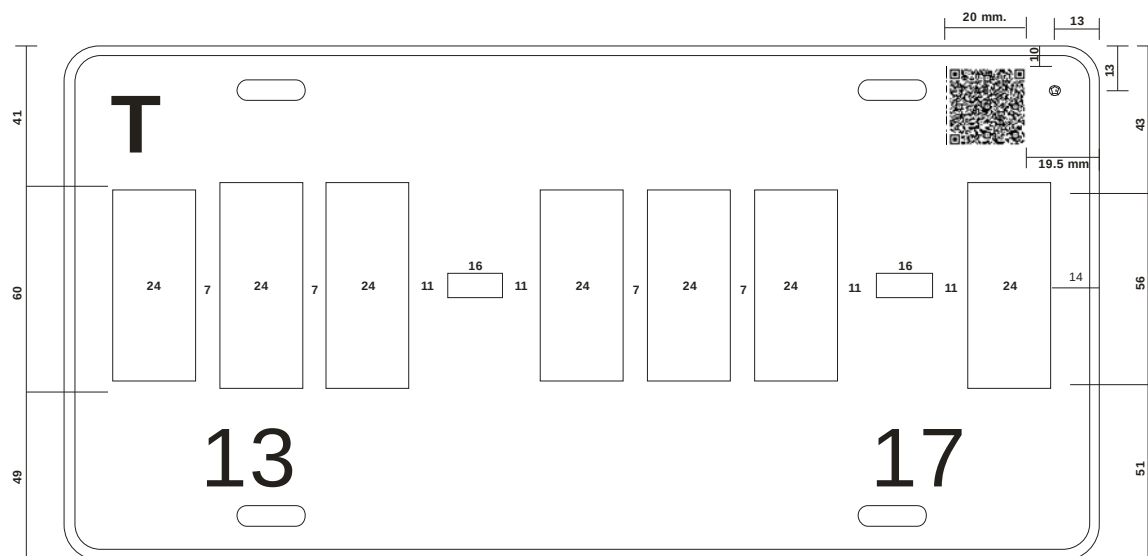
Figura 21 Separación de caracteres (letras y dígitos) placas con siete caracteres y guiones Placa para TRANSPORTE PRIVADO REMOLQUE (Entidades Federativas)
