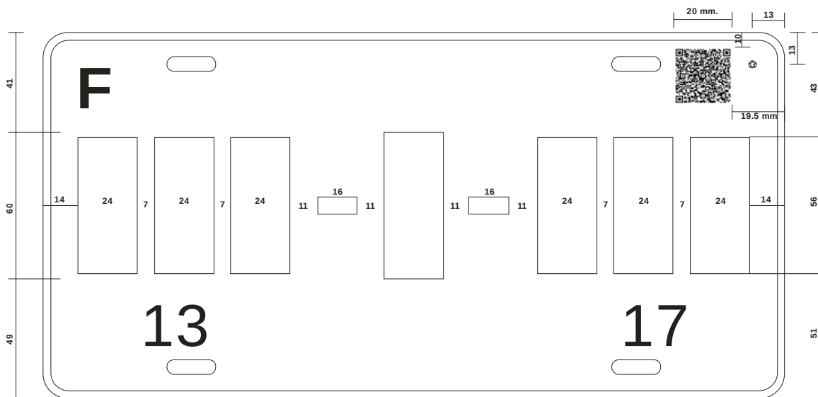
Figura 23 Separación de caracteres (letras y dígitos) placas con siete caracteres y guiones Placa para Servicio Público Local; Distrito Federal; Con itinerario fijo
