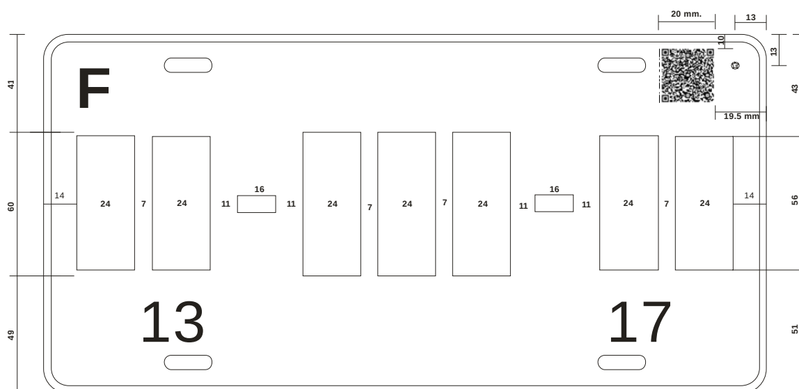
Figura 20 Separación de caracteres (letras y dígitos) placas con siete caracteres y guiones Placa para TRANSPORTE PRIVADO AUTOBÚS (Entidades Federativas)
