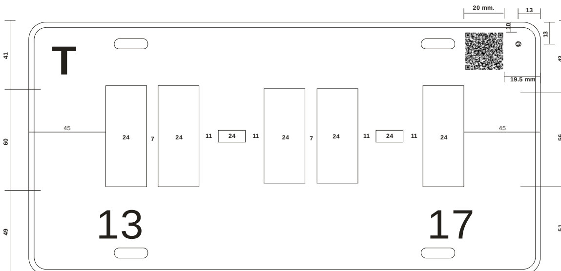
Figura 17 Separación de caracteres (letras y dígitos) placas con cinco caracteres y guiones Placa para TRANSPORTE PRIVADO REMOLQUE (Distrito Federal)
