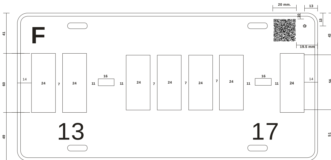
Figura 19 Separación de caracteres (letras y dígitos) placas con siete caracteres y guiones Placa para TRANSPORTE PRIVADO CAMIÓN (Entidades Federativas)
