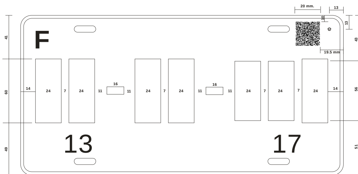
Figura 34 Separación de caracteres (letras y dígitos) placa con siete caracteres y guiones Placa para vehículos del H. CUERPO DE BOMBEROS de las Entidades Federativas
