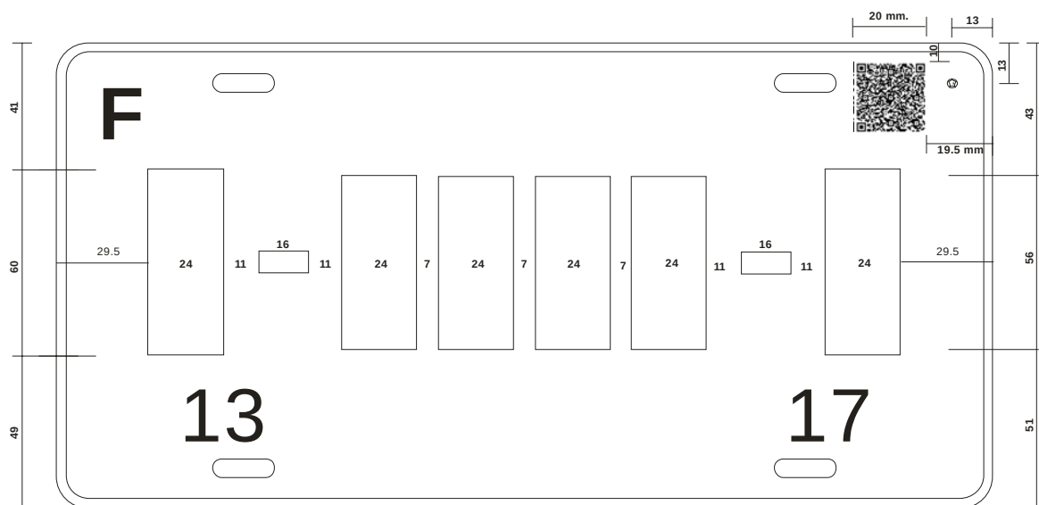
Figura 4 Separación de caracteres (letras y dígitos) placas con seis caracteres y guiones Para el servicio de autotransporte federal PASAJE ECONÓMICO MIXTO (Midibús)
