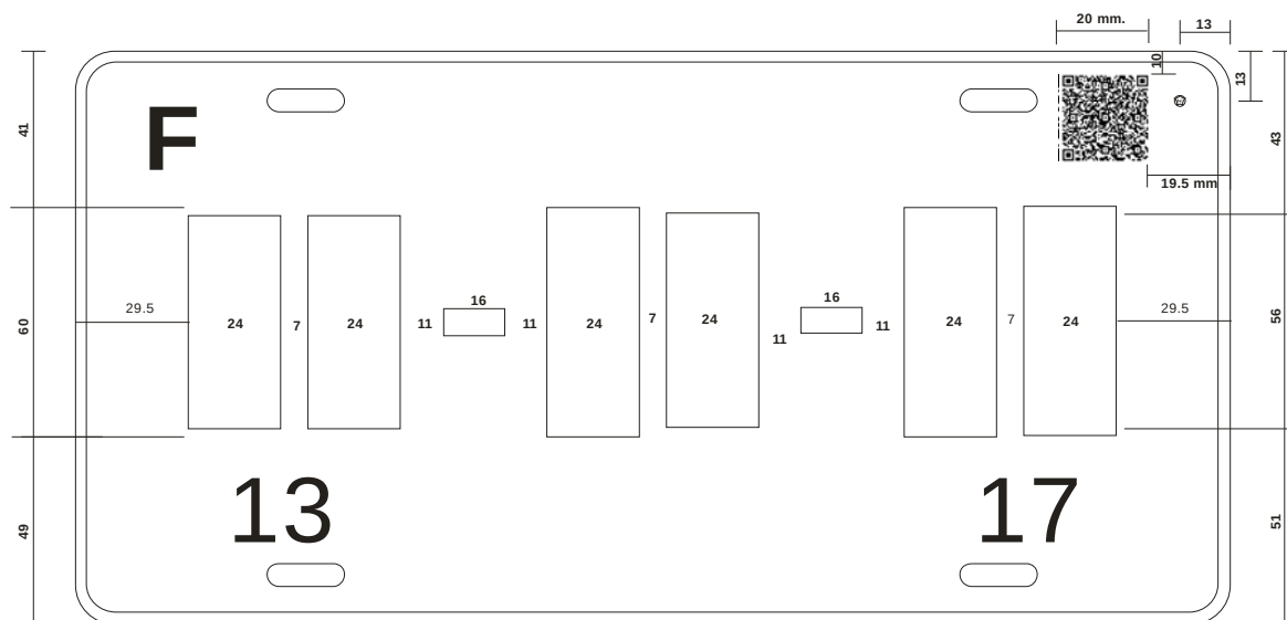
Figura 5 Separación de caracteres (letras y dígitos) placas con seis caracteres y guiones Para el servicio de autotransporte federal TRASLADO NACIONAL (Para todo tipo de vehículo)
