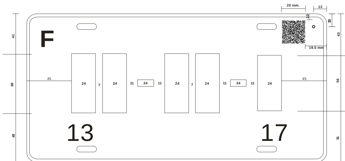
Figura 12 Separación de caracteres (letras y dígitos) placas con cinco caracteres y guiones Placa para DEMOSTRACIÓN (Distrito Federal)
