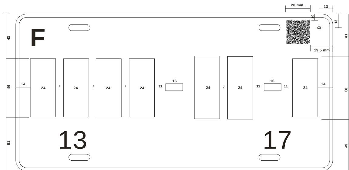
Figura 15 Separación de caracteres (letras y dígitos) placas con siete caracteres y guiones Placa para CAMIÓN (Distrito Federal)
