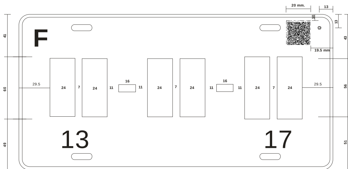
FIGURA 6.- Separación de caracteres (letras y dígitos) placas con seis caracteres Para el servicio de autotransporte federal PAQUETRIA Y MENSAJERIA
