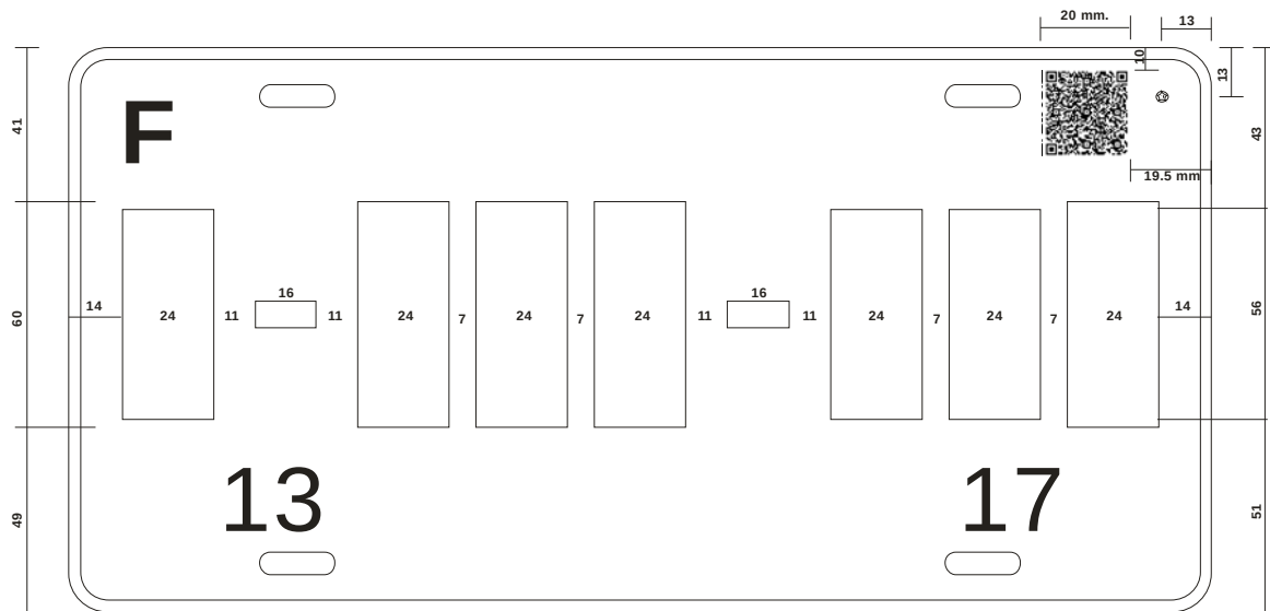
Figura 26 Separación de caracteres (letras y dígitos) placas con siete caracteres y guiones Placa para Camión Público Local (Entidades Federativas)
