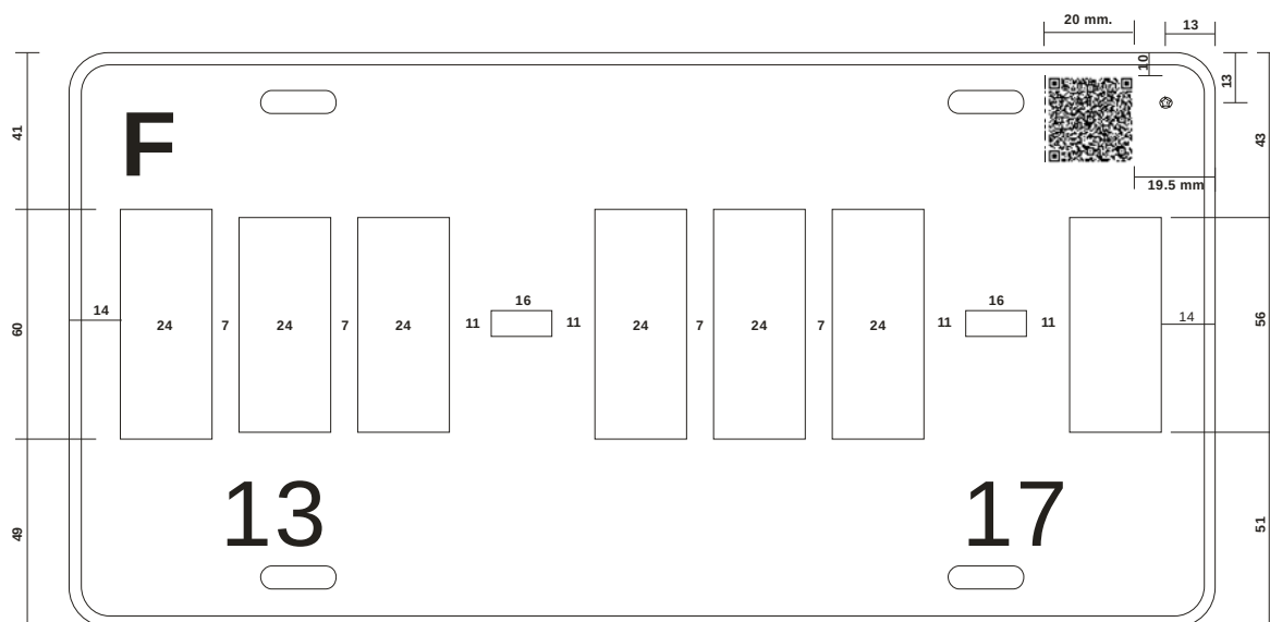
Figura 8 Separación de caracteres (letras y dígitos) placas con siete caracteres y guiones Para TRANSPORTE PRIVADO AUTOMÓVIL FRONTERIZO
