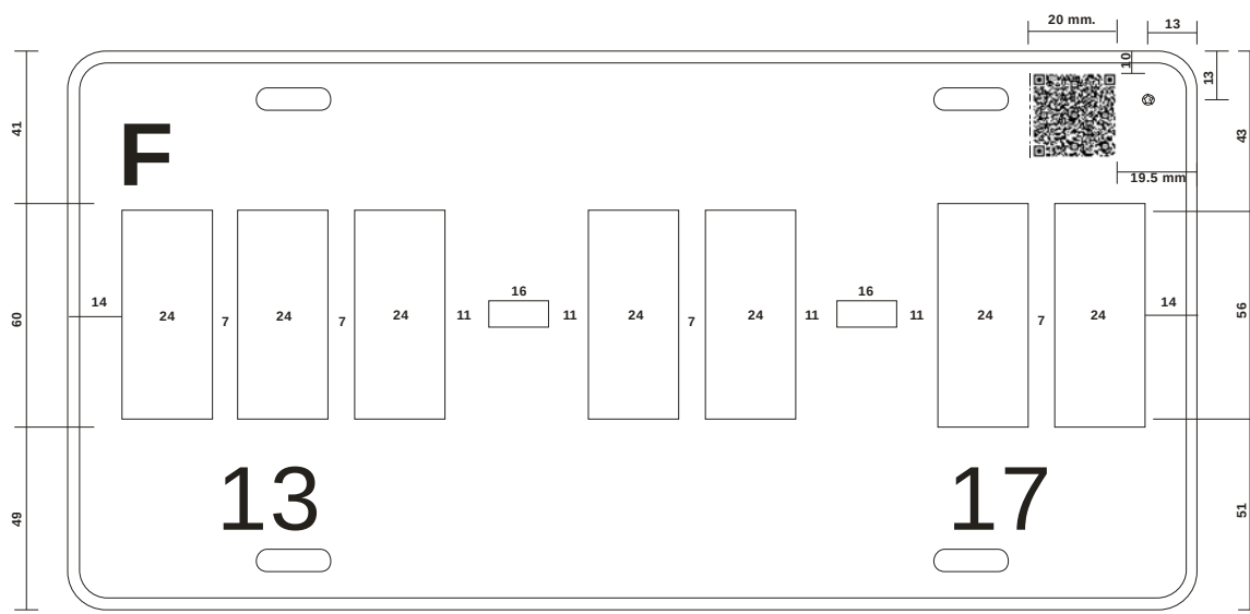
Figura 9 Separación de caracteres (letras y dígitos) placas con siete caracteres y guiones Placa para CAMIÓN, AUTOBÚS y REMOLQUE del TRANSPORTE PRIVADO FRONTERIZO
