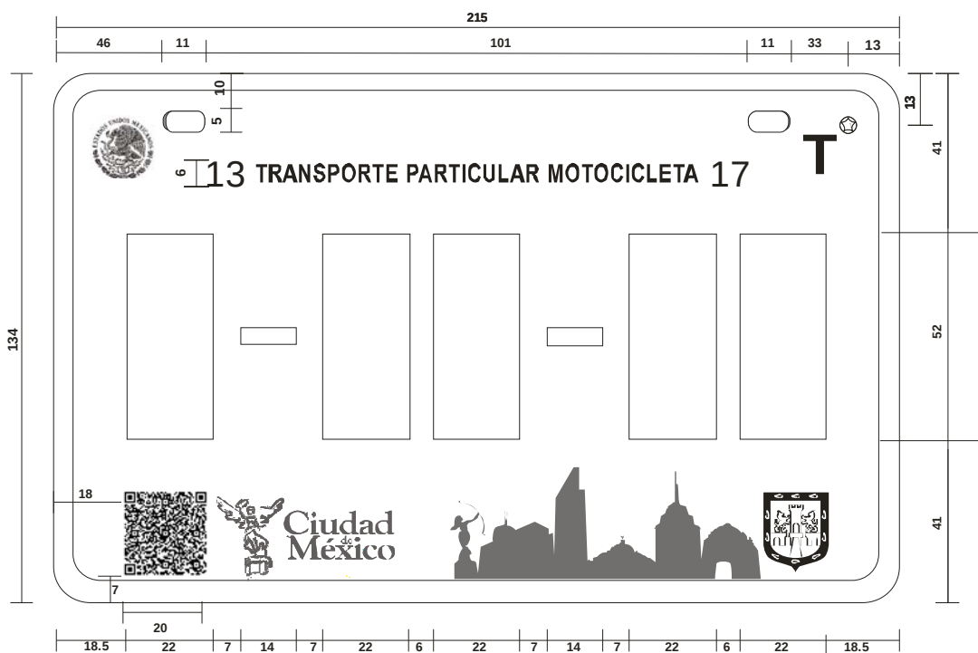
Figura 29 Separación de caracteres (letras y dígitos) placas con cinco caracteres y guiones MODELO DE PLACA PARA EL DISTRITO FEDERAL Y ENTIDADES FEDERATIVAS
