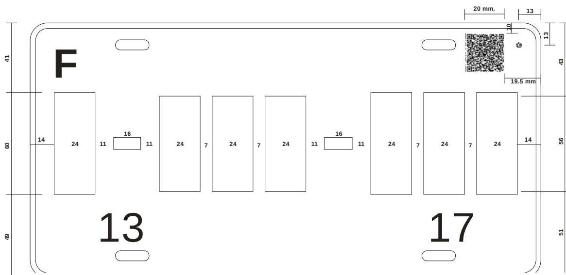
Figura 14 Separación de caracteres (letras y dígitos) placas con siete caracteres y guiones Placa para AUTOMÓVIL (Distrito Federal)
