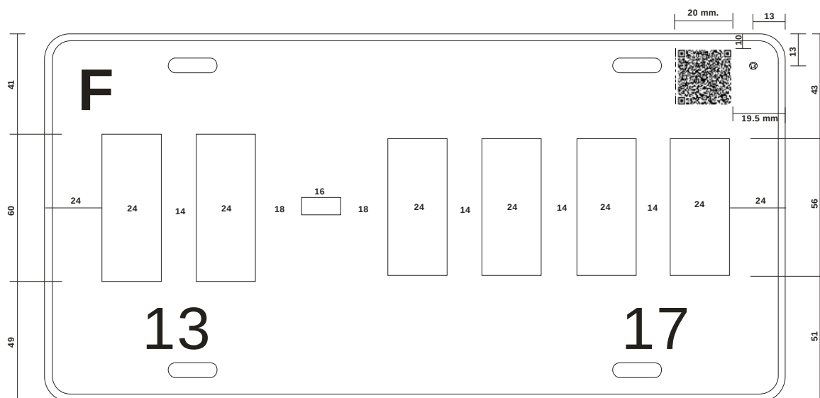
Figura 22 Separación de caracteres (letras y dígitos) placas con seis caracteres y guiones Placa para Servicio Público Local; Distrito Federal; Libre y Sitio
