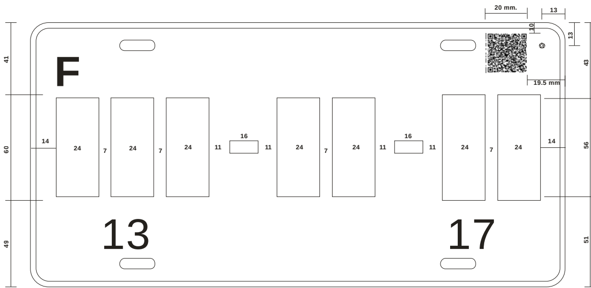
Figura 27 Separación de caracteres (letras y dígitos) placas con siete caracteres y guiones Placa para Autobús Público Local (Entidades Federativas)
