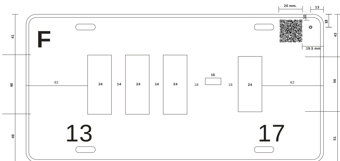
Figura 35 Separación de caracteres (letras y dígitos) placa con cuatro caracteres y guión Placa para vehículos de INSPECTOR DE VÍAS GENERALES DE COMUNICACIÓN de la Secretaría de Comunicaciones y Transportes
