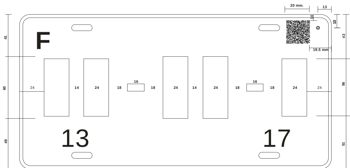
Figura 16 Separación de caracteres (letras y dígitos) placas con cinco caracteres y guiones Placa para TRANSPORTE PRIVADO AUTOBÚS (Distrito Federal)
