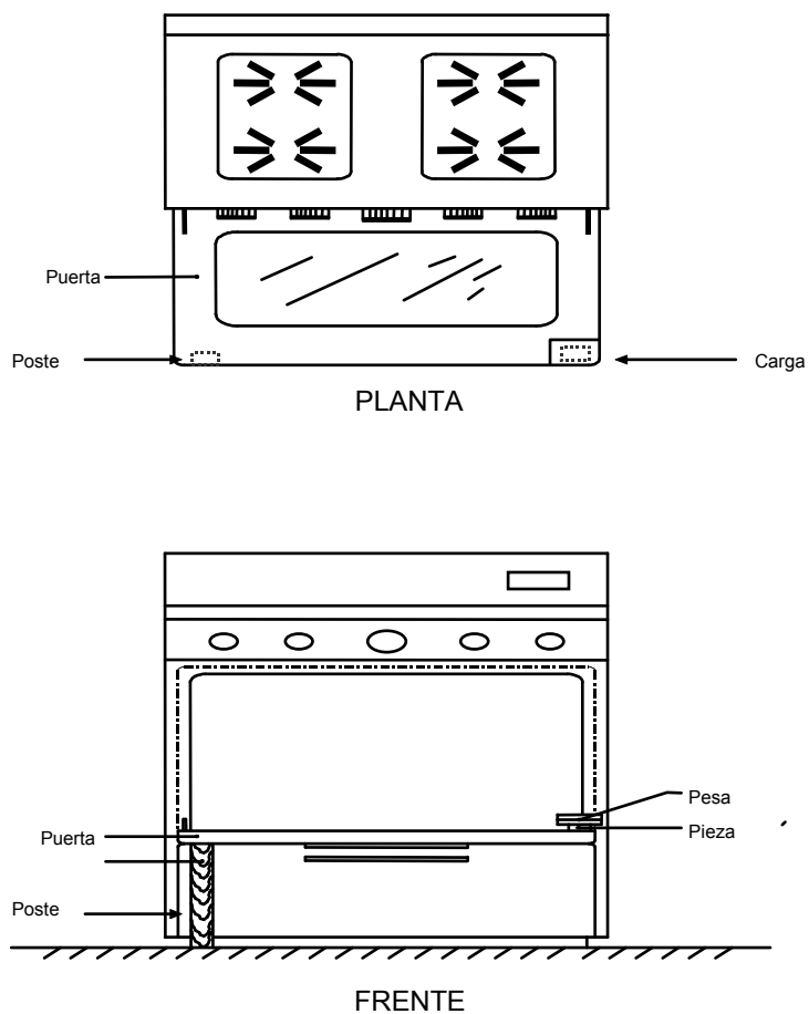
Figura 1. Pruebas de resistencia a masas sobre una esquina de la puerta que se abre hacia abajo (ilustrativa mas no limitativa)
