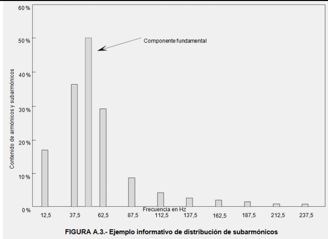
FIGURA A.3.- Ejemplo informativo de distribución de subarmónicos
