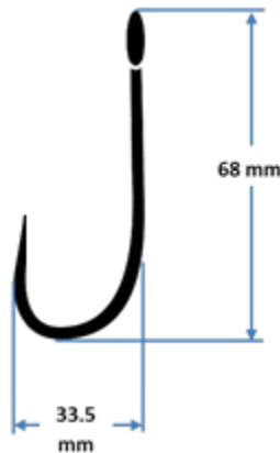
Fig. 1.- Dimensiones mínimas de anzuelos atuneros
