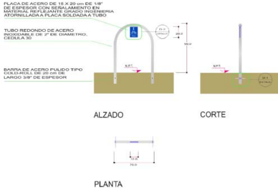
Gráfico 2: Detalle del mueble bici estacionamiento tipo "U invertida"
