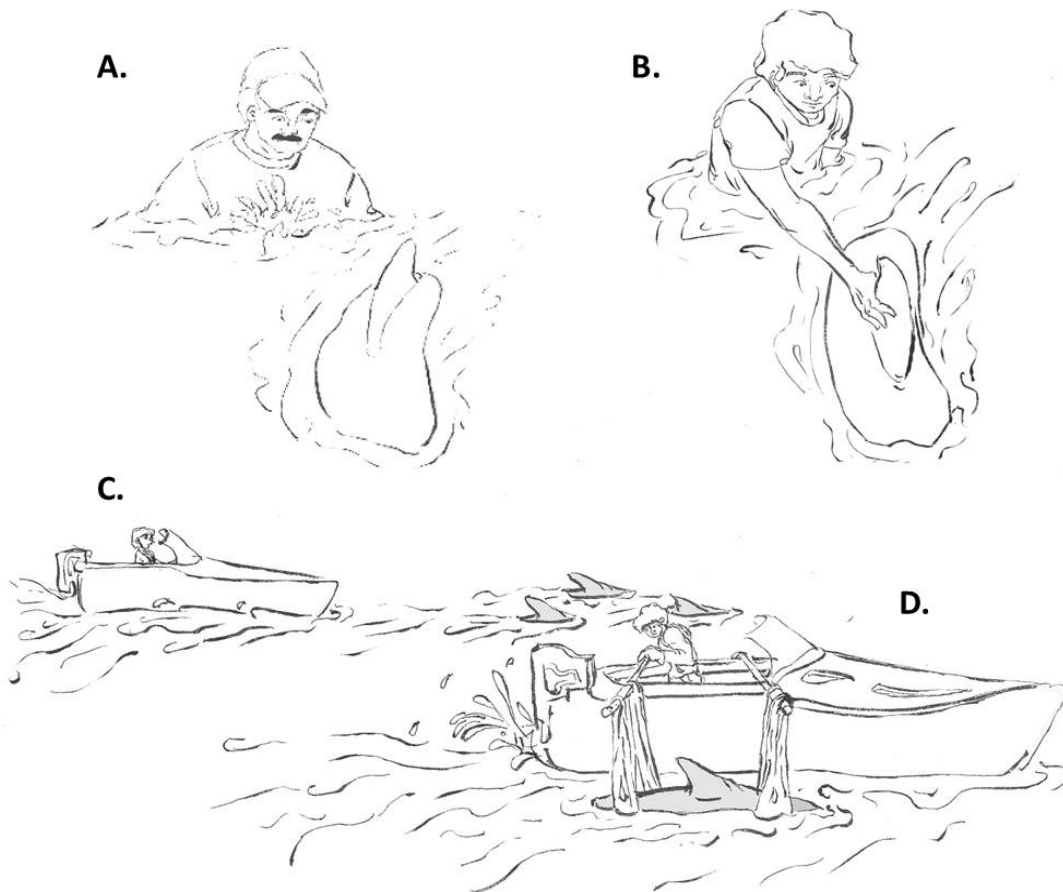
Figura 1. Técnicas para prevenir el varamiento y regresar los cetáceos al mar. Las técnicas para prevenir los varamientos y regresar a los cetáceos al mar, incluyen el uso de ruido subacuático, la reorientación manual, el arreo mediante una embarcación pequeña y el remolque en un cabestrillo o camilla.
