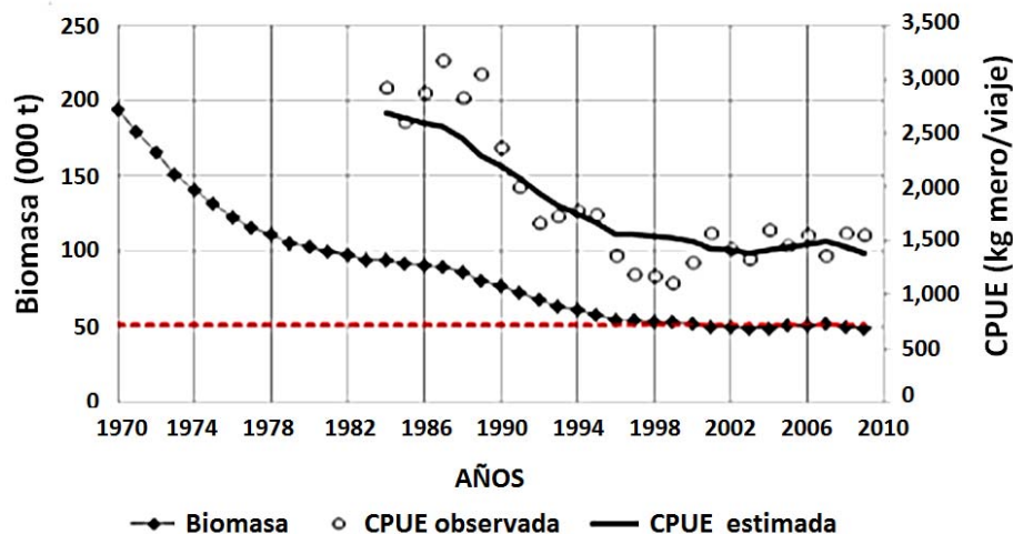
Figura 17. Ajuste del modelo dinámico de Schaefer a los datos de captura por unidad de esfuerzo (CPUE) observados y estimados y biomasa estimada para el mero rojo ( Epinephelus morio ) capturado por la flota yucateca de mediana altura, en el Banco de Campeche; el punto de referencia límite (PRL), consiste en que la biomasa en el 2009 no sea menor a la biomasa promedio estimada en los últimos 15 años ( B_{1995-2009} = 52,000 t).
