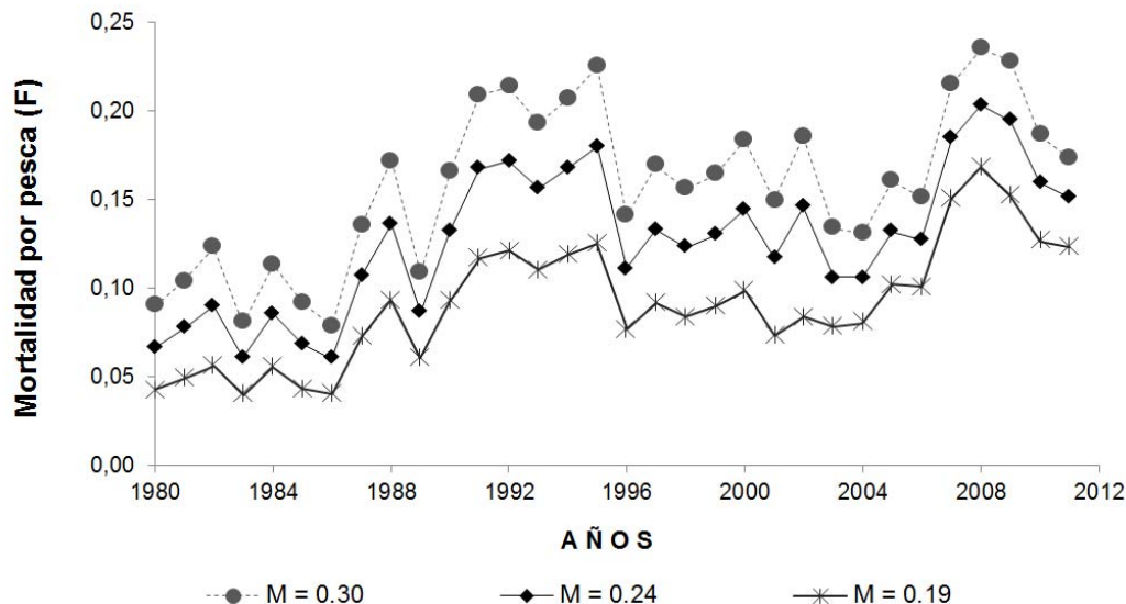
Figura 19. Comportamiento anual de la mortalidad por pesca ( F año -1 ) registrada en la pesquería de mero rojo ( Epinephelus morio ), en el Banco de Campeche, considerando tres valores anuales de mortalidad natural ( M ).
