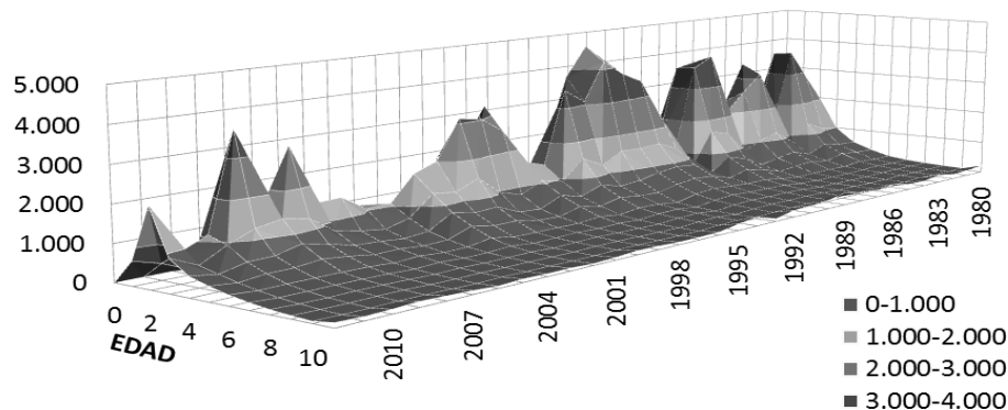
Figura 18. Estructura de la captura por clase de edad del mero rojo ( Epinephelus morio ) (1980-2012, registrada en el Banco de Campeche por las flotas mexicanas (artesanal y de mediana altura).
