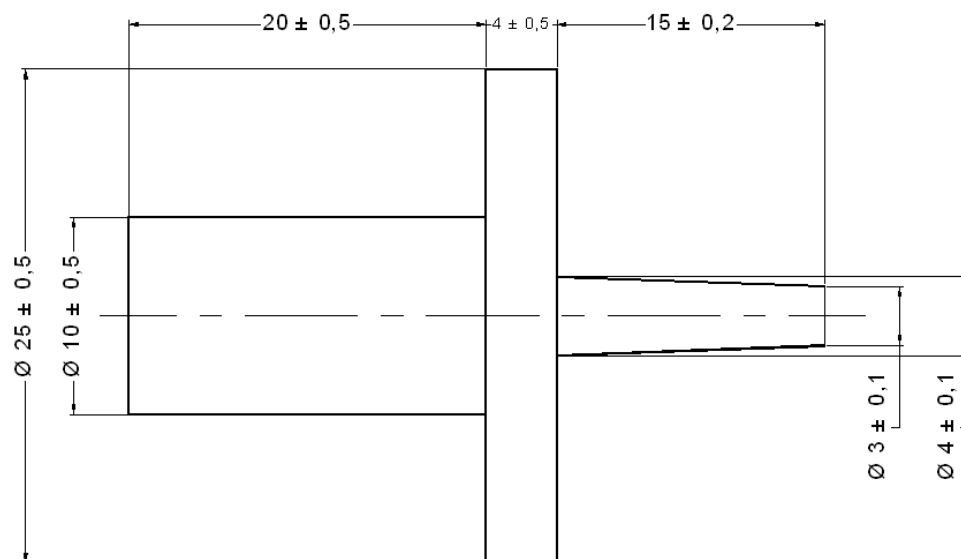
Figura 3. Aguja de prueba
