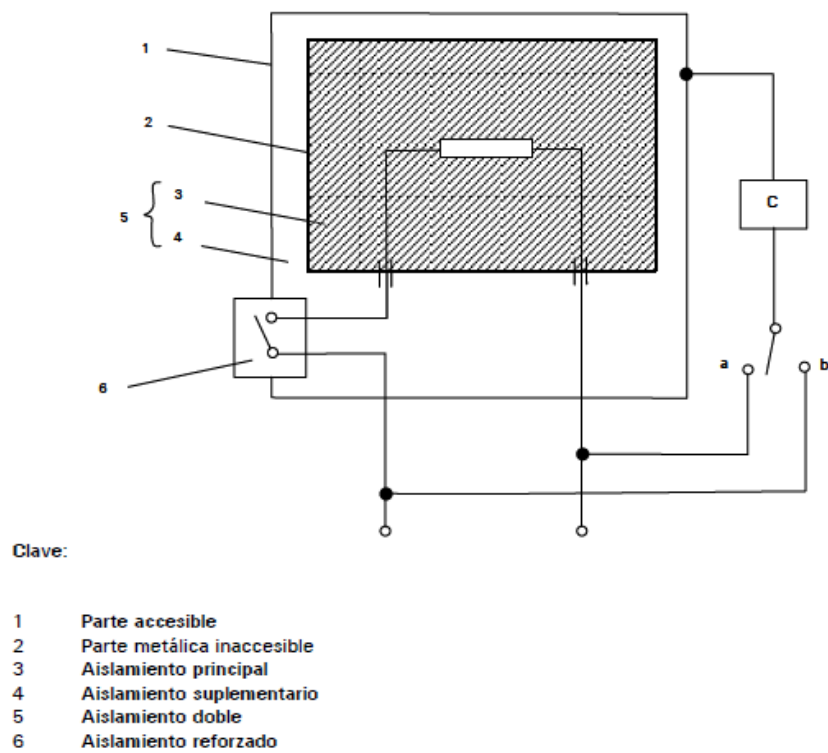
Figura 5. Diagrama para la medición de corriente de fuga a la temperatura de operación para equipos monofásicos Clase II
