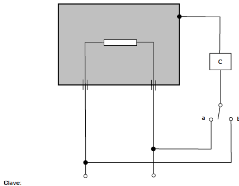
Figura 6. Aparatos distintos de Clase II monofásicos
